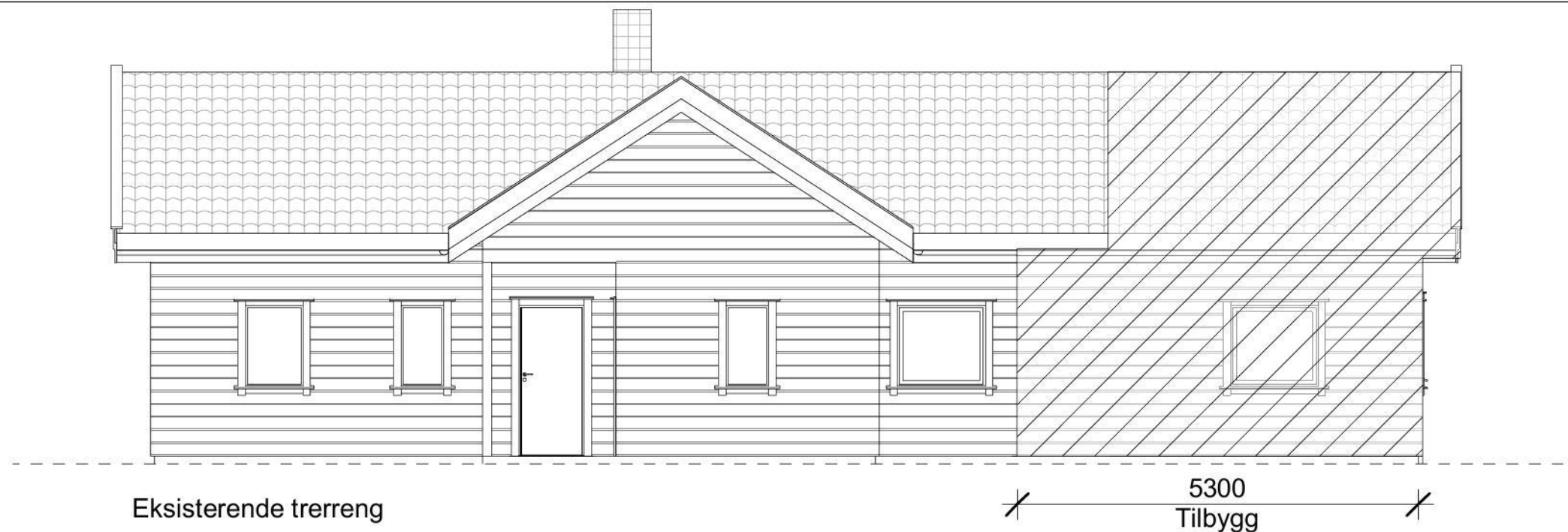
Fasade mot Sør 1 : 100
