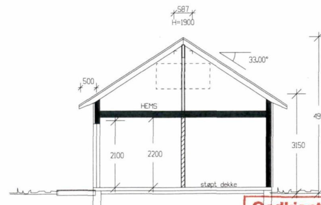
Snitt A-A
