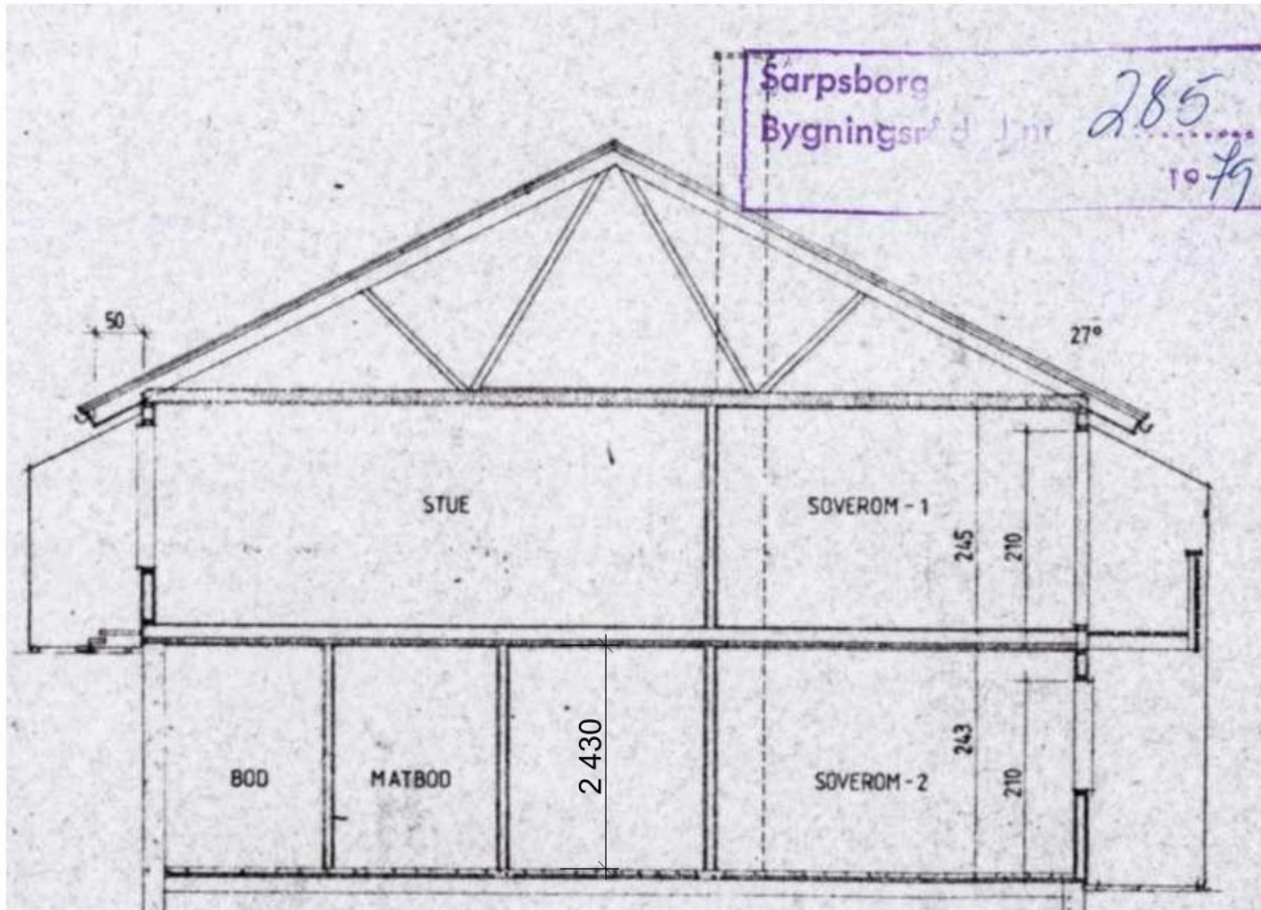
Typisk Snitt 1:100
