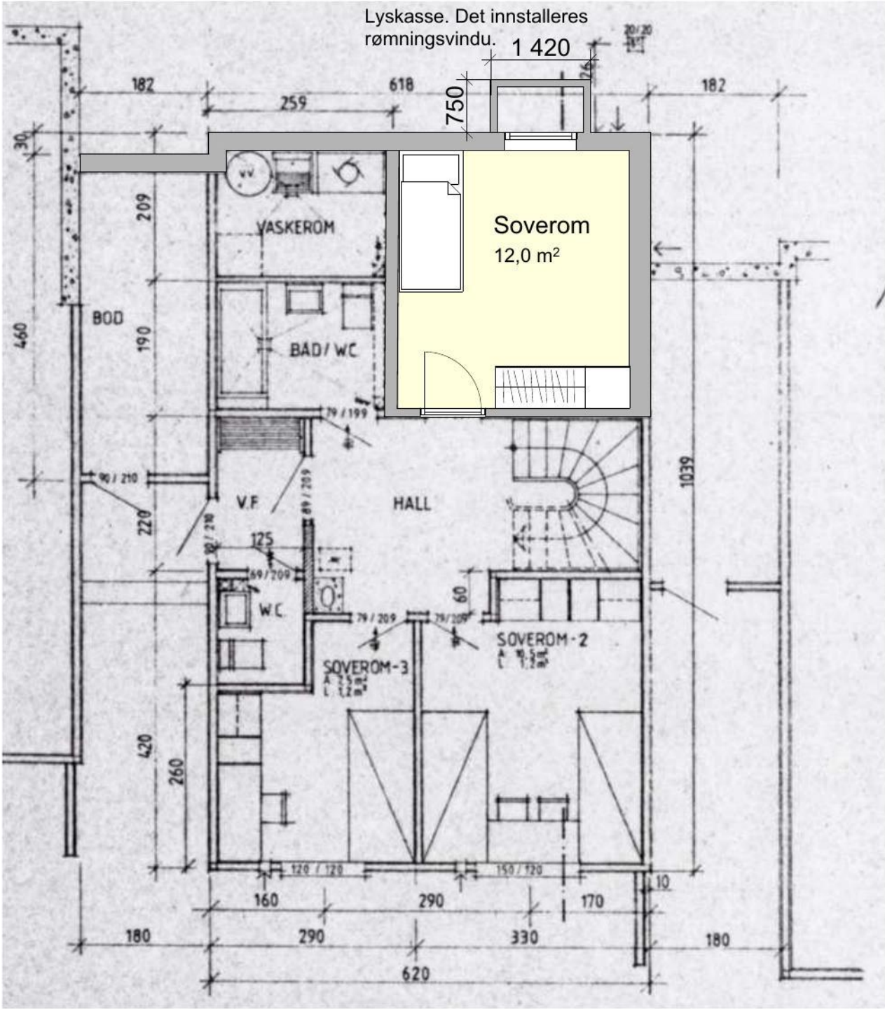
Plan U.etg 1:100
