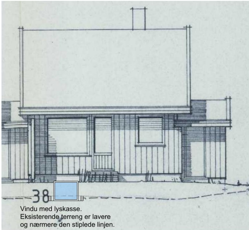
Fasade Vest 1:100
