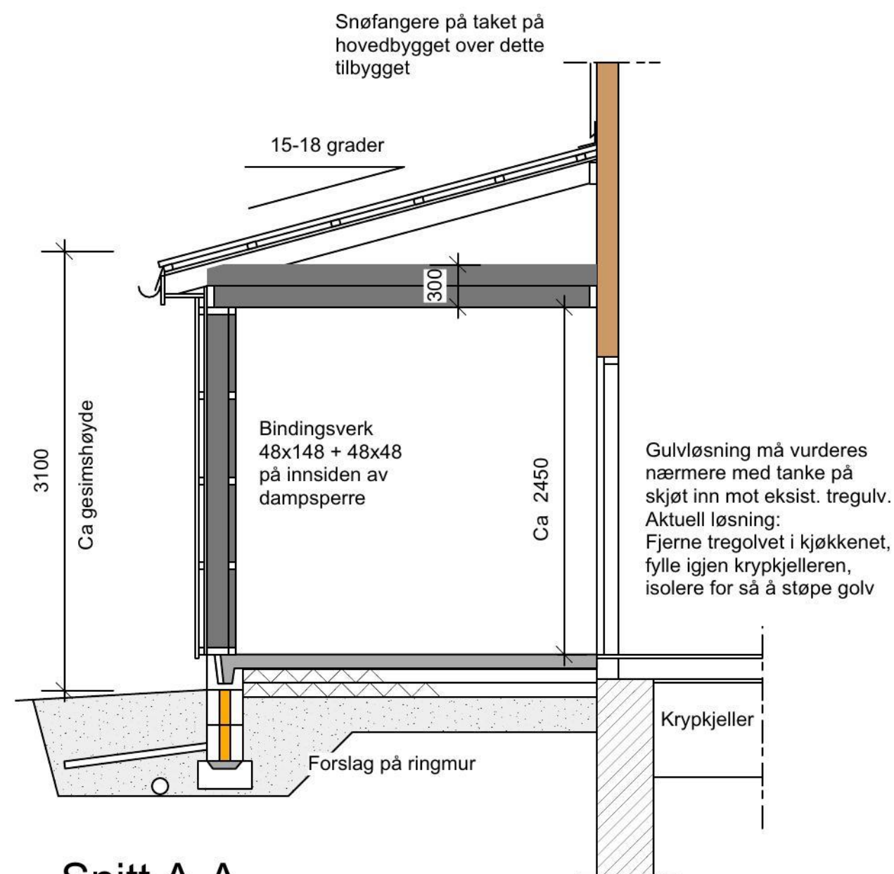
Snitt A-A Mål 1:50
