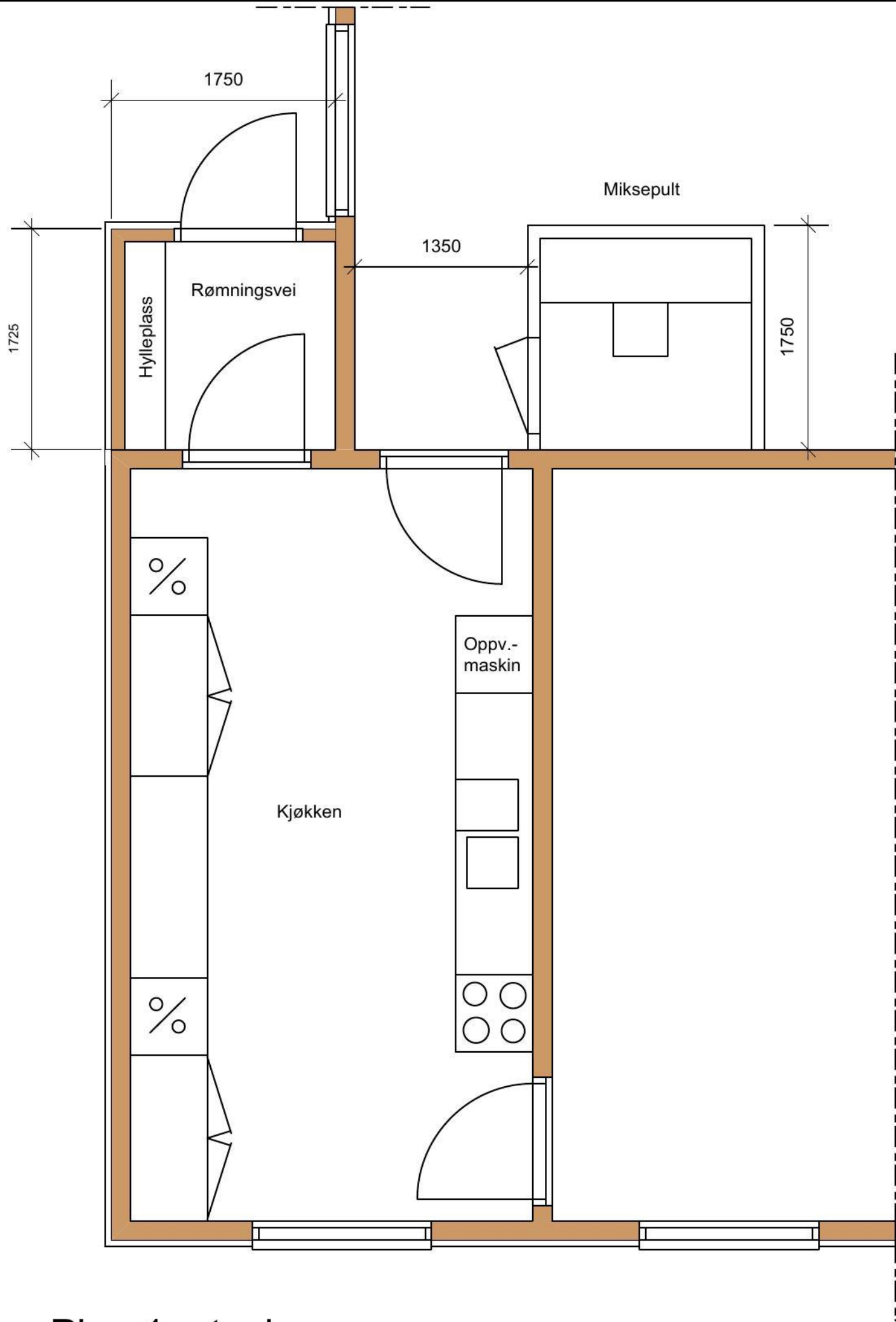
Plan 1. etasje Eksisterende løsning Mål 1:50
