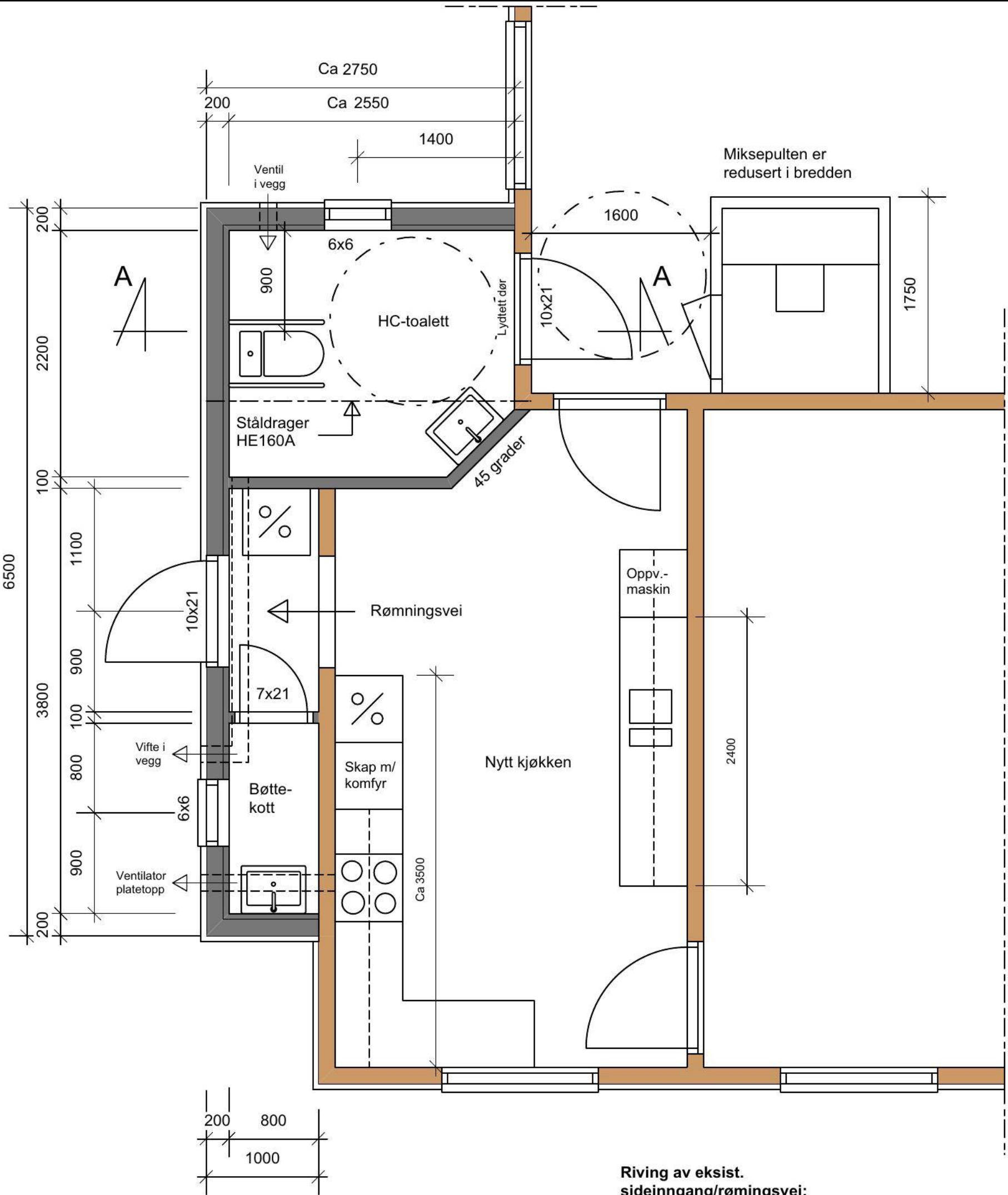
Plan 1. etasje Tilbygg/ombygging Mål 1:50
