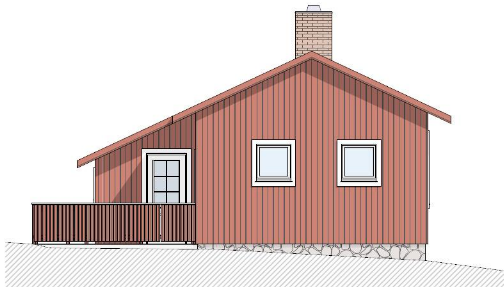
Fasade Øst
