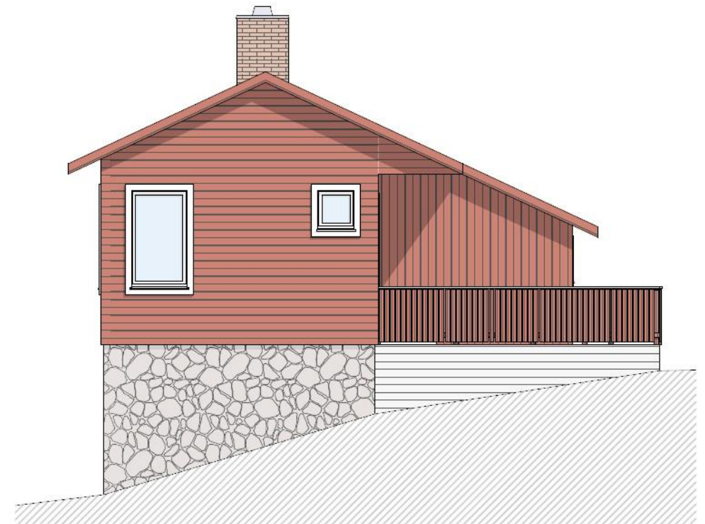
Fasade Vest
