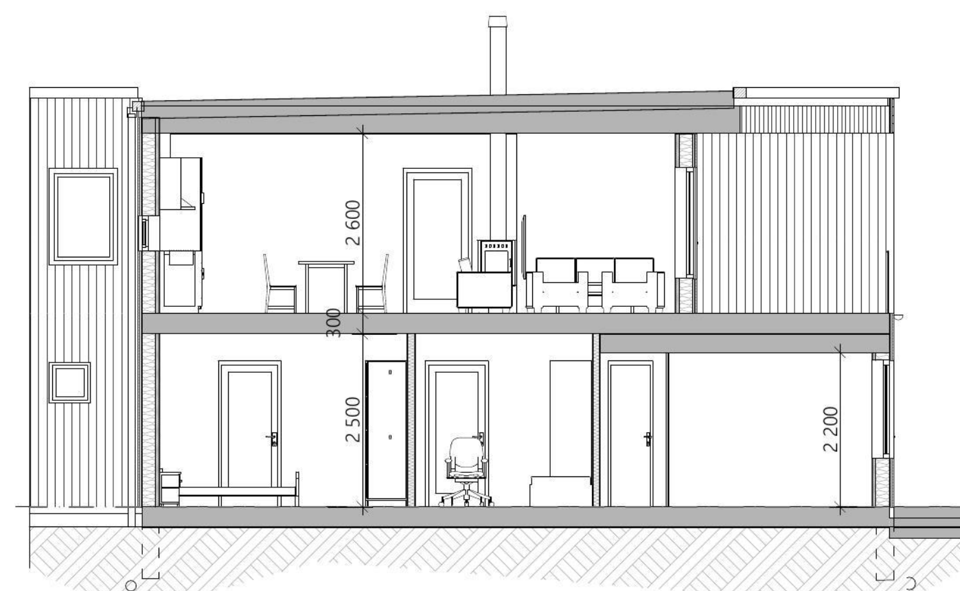
Snitt C
