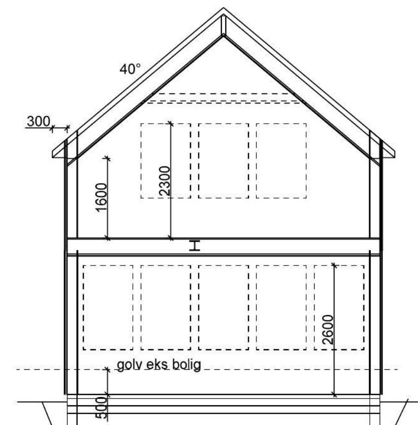
SNITT B-B
