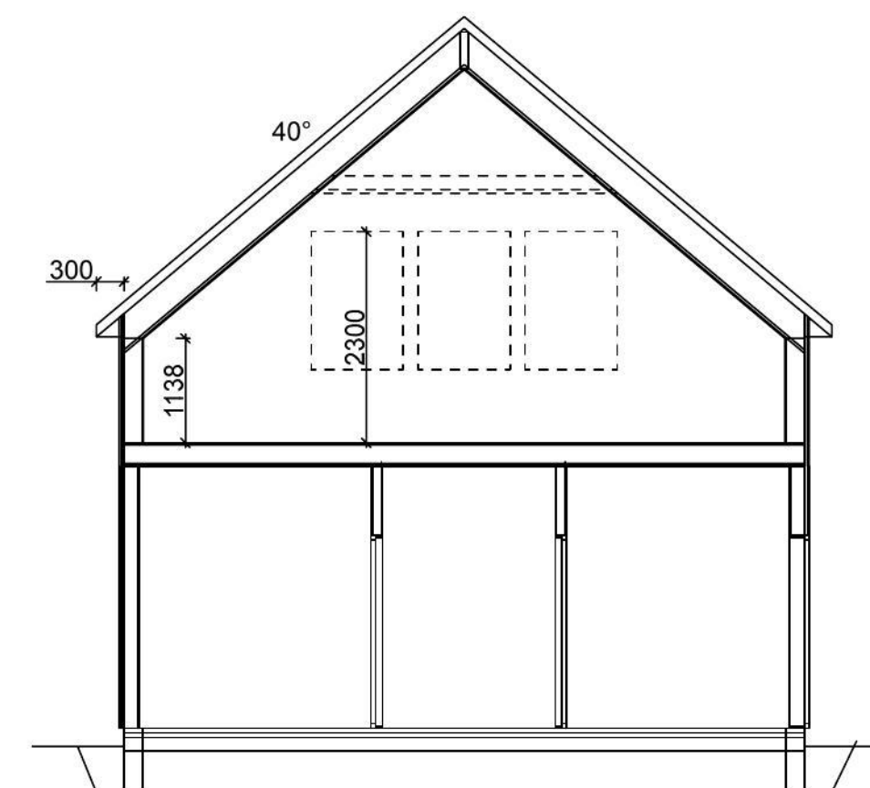
SNITT C-C
