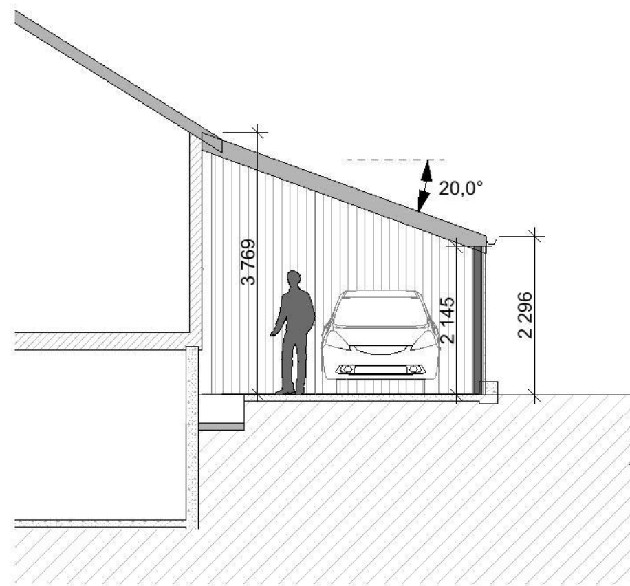
Snitt A 1:100
