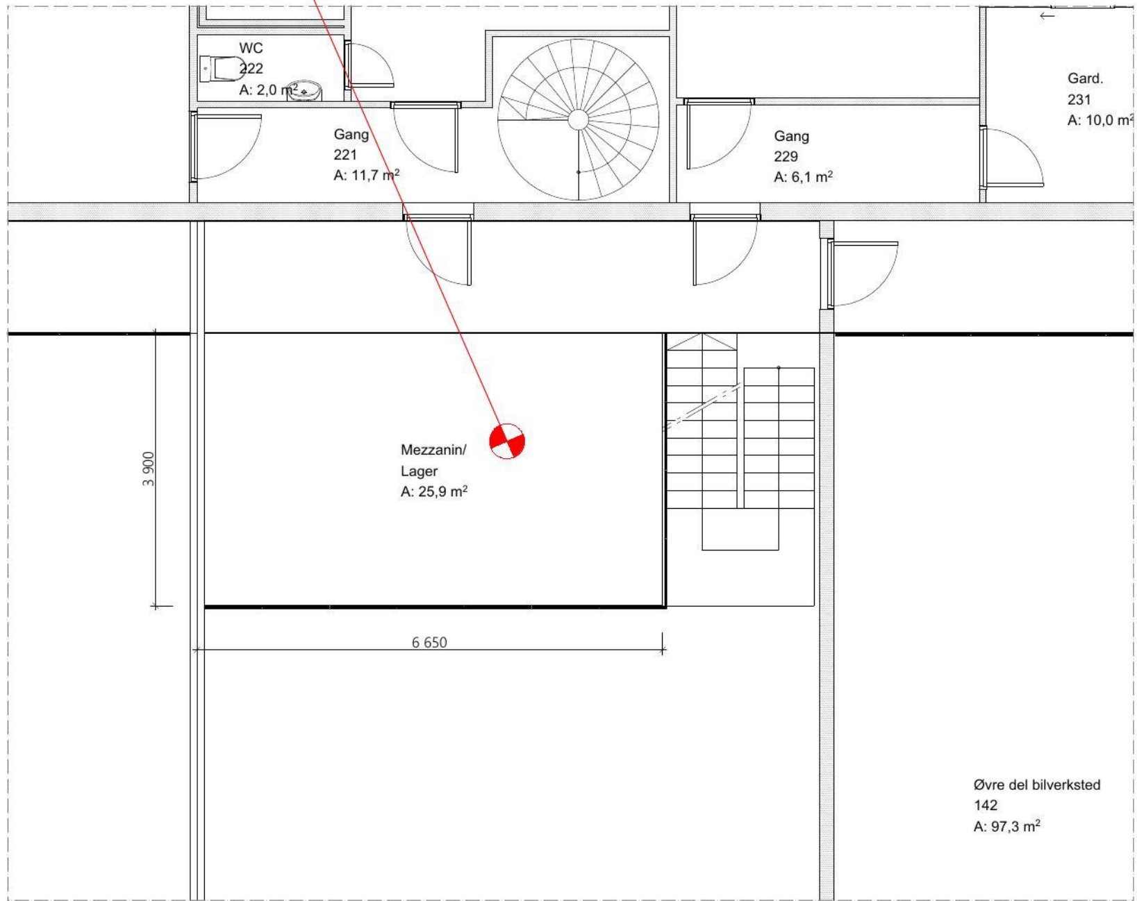
1:100 Ny mezzanin
