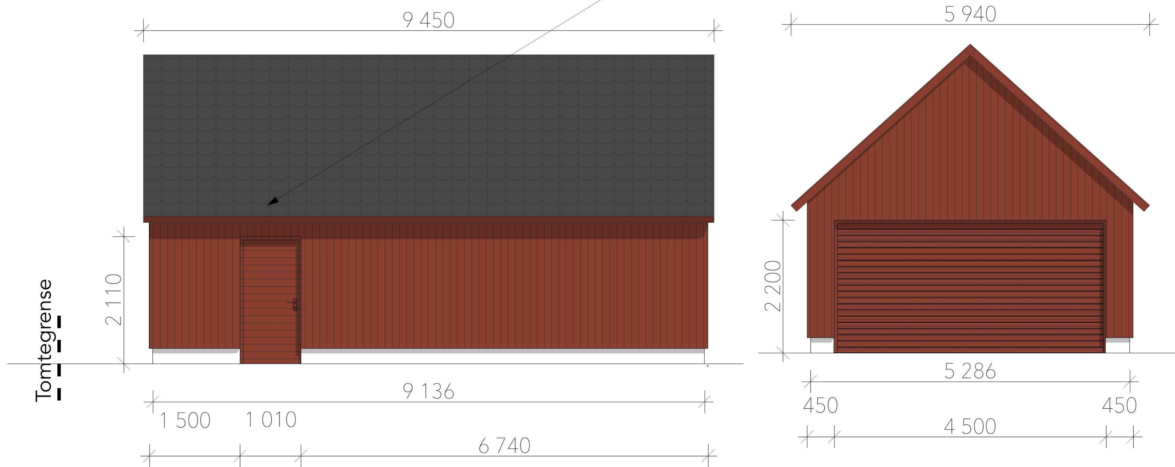
1:50 Fasade Sør
