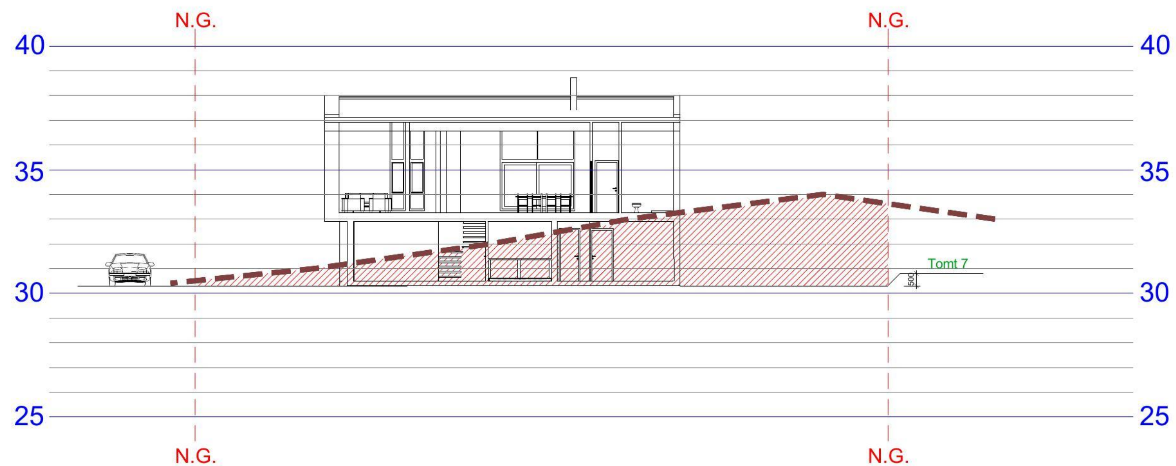
Snitt b-b
