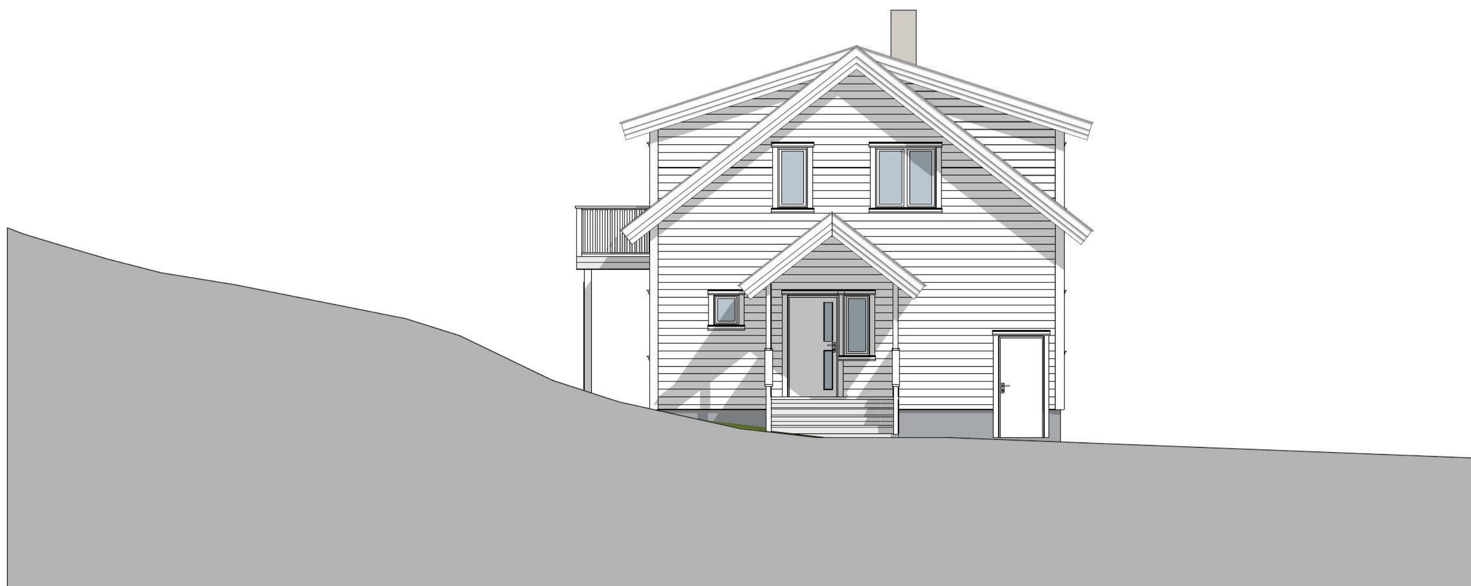
1:100 Fasade Nord
