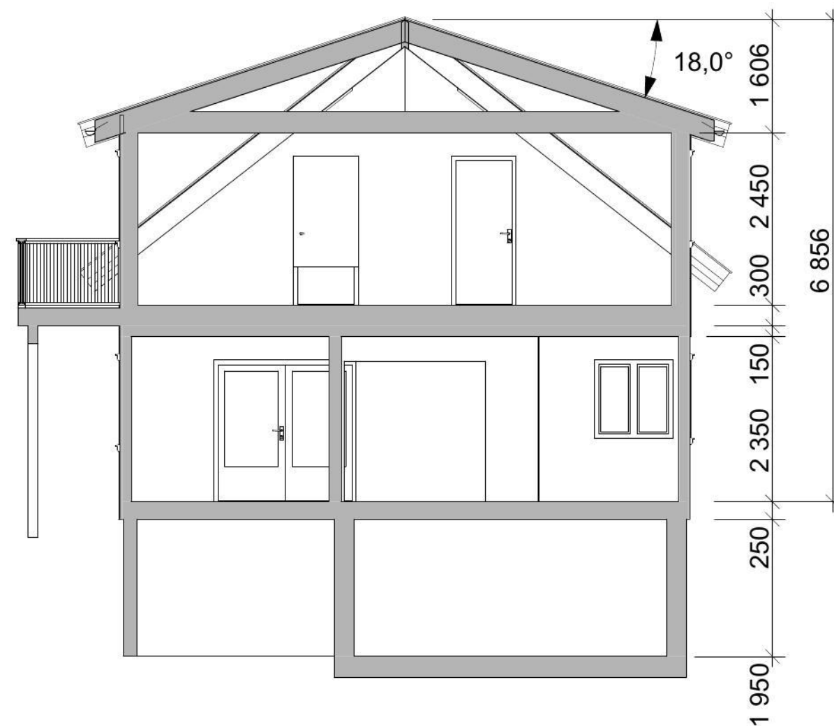
1:100 Snitt B
