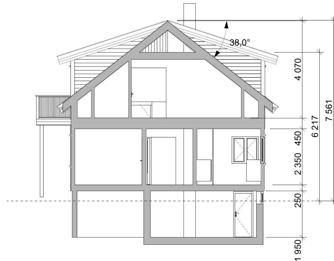
1:100 Snitt A
