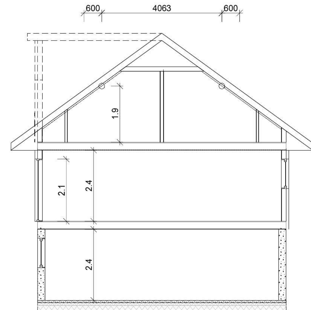
Snitt A-A
