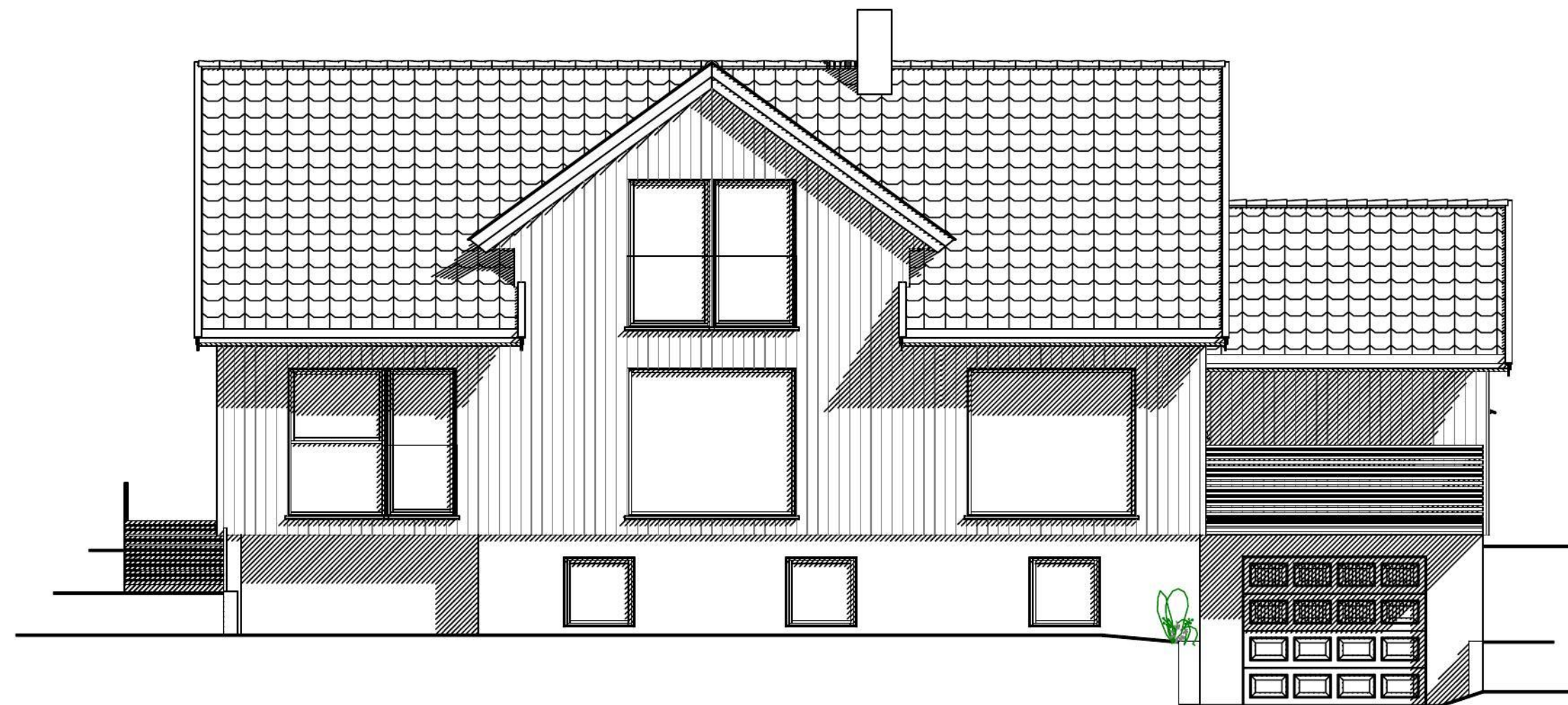
Fasade Vest
