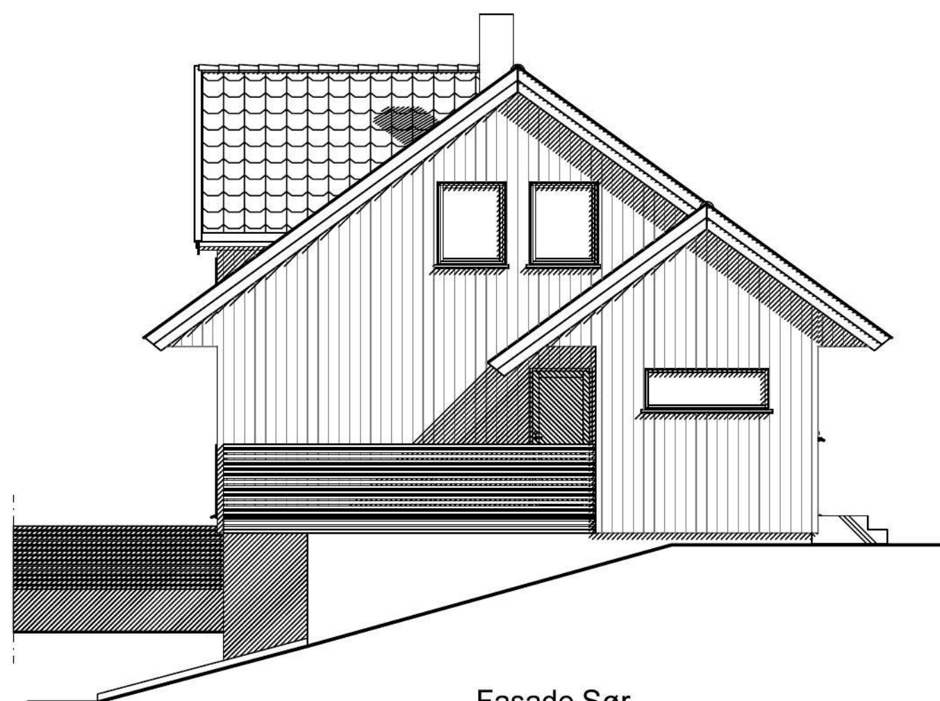
Fasade Sør
