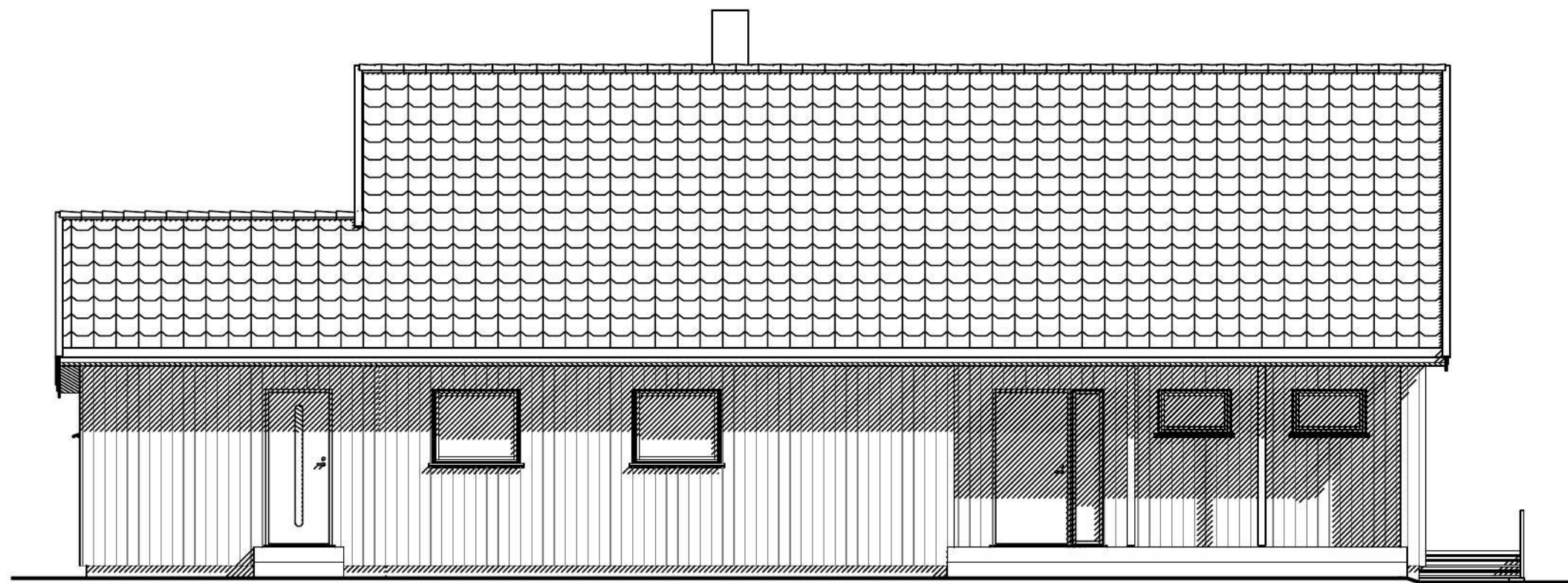
Fasade Øst
