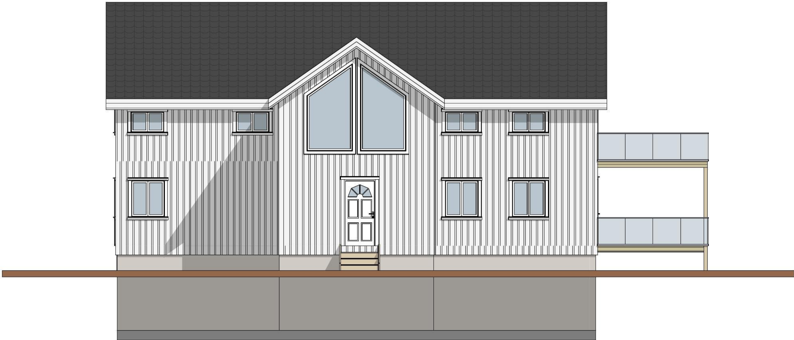
1:100 Fasade Øst
