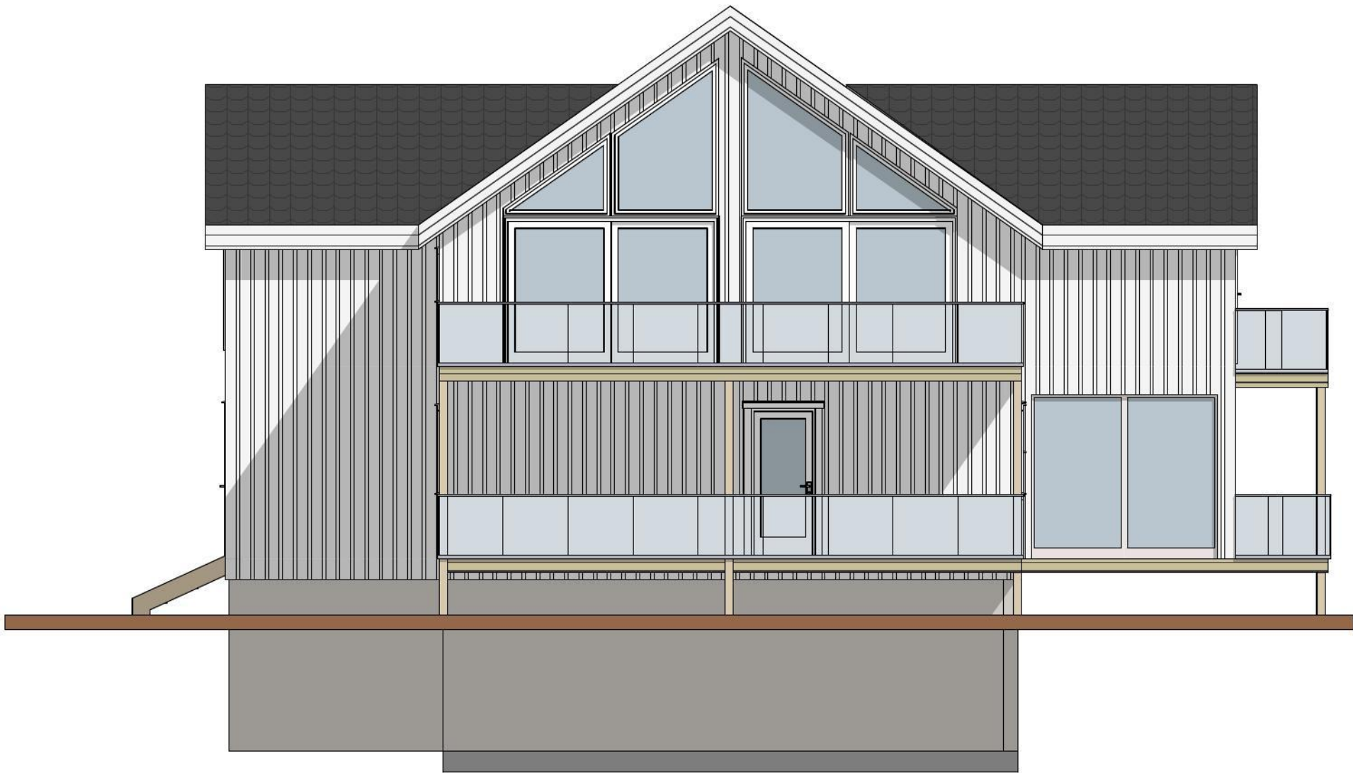
1:100 Fasade Nord
