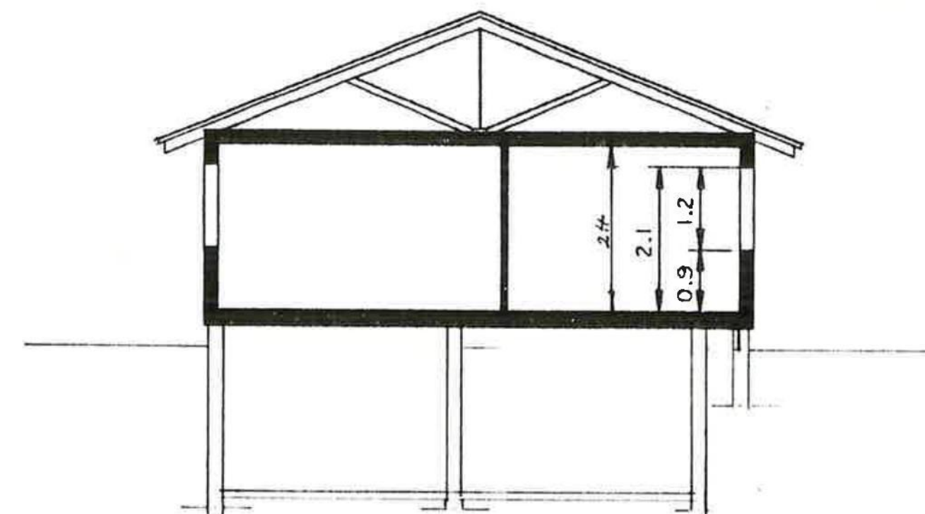
SNITT
