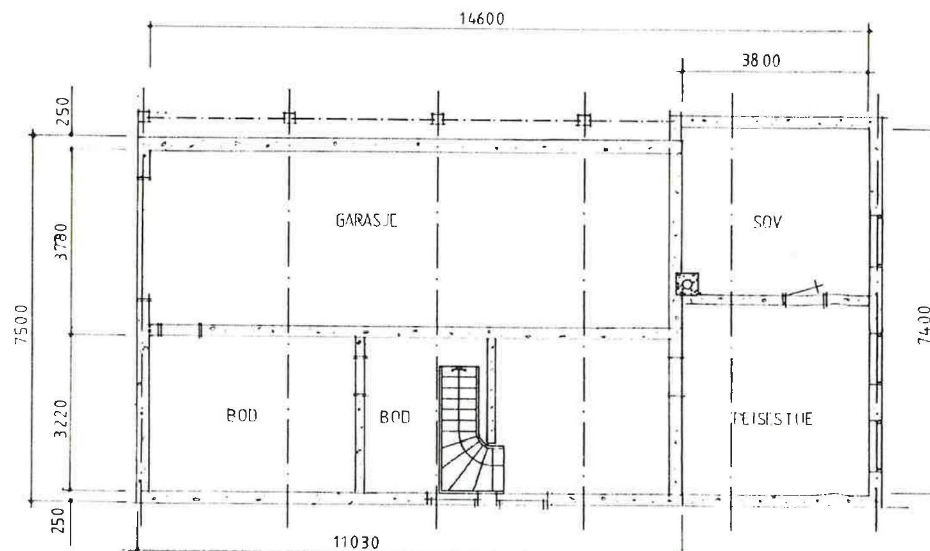
MIDLERTIDIG FUNDAMENTPLAN MÅ IKKE BENYTTES SOM ARBEIDSTEGNING
