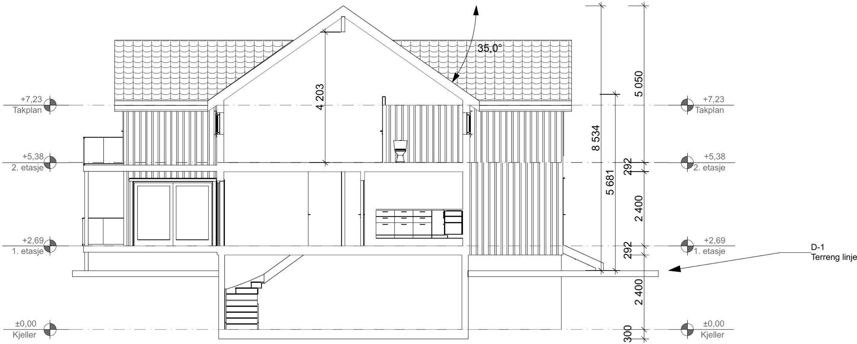
1:100 Snitt A
