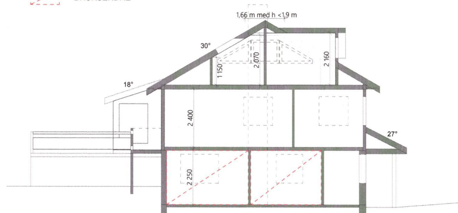
Snitt 1:100
