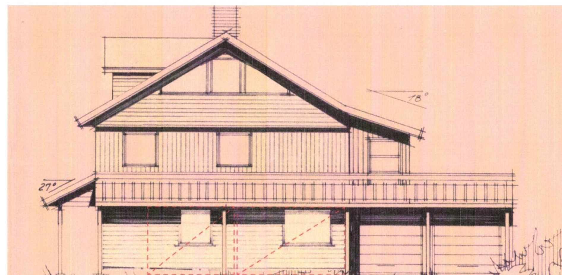
Fasade Nord 1:200
