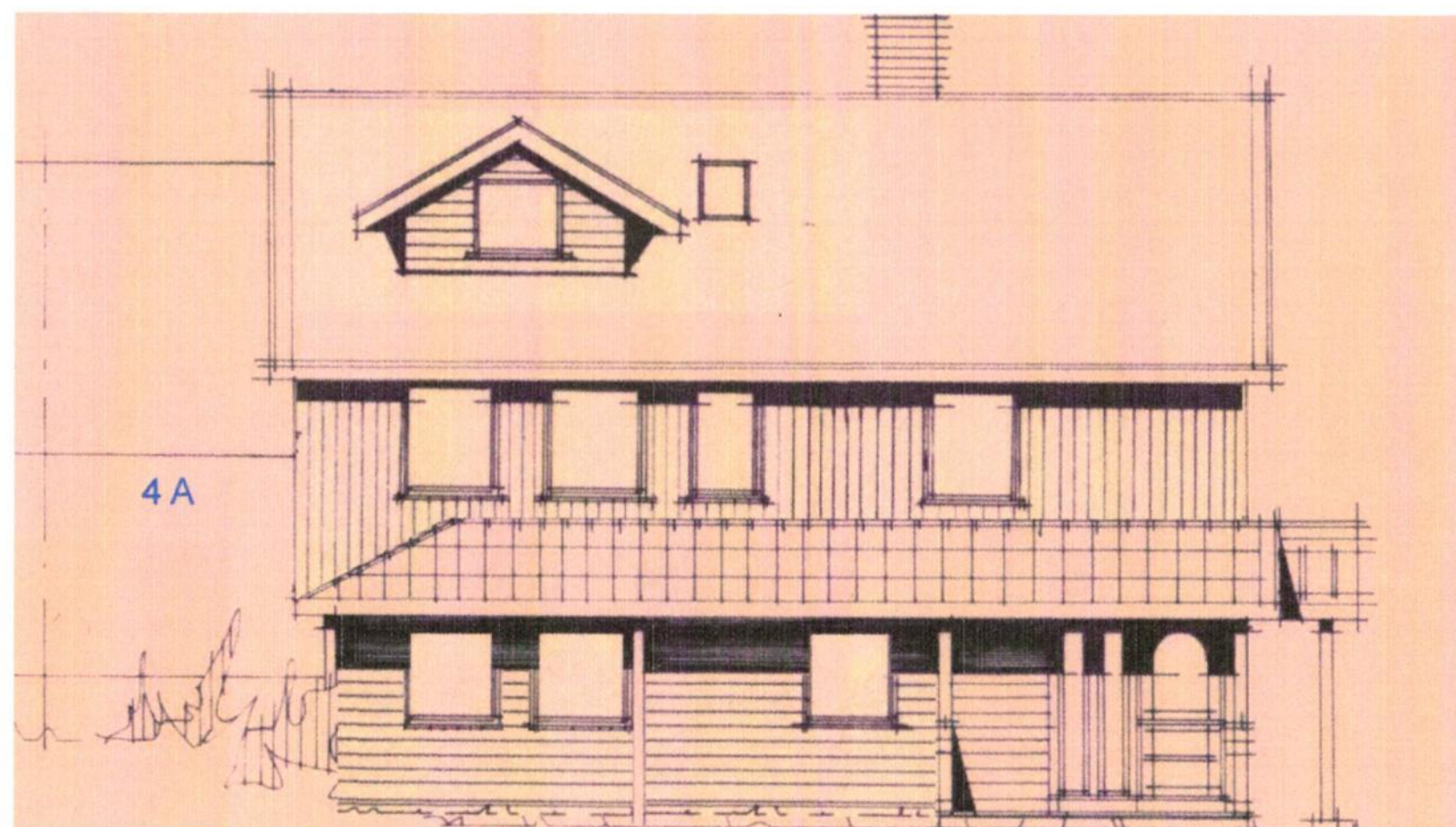
Fasade Øst 1:200
