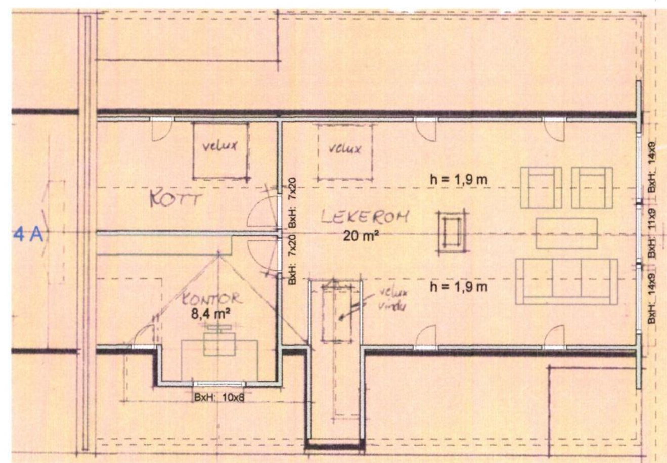
Plan Loft 1:100
