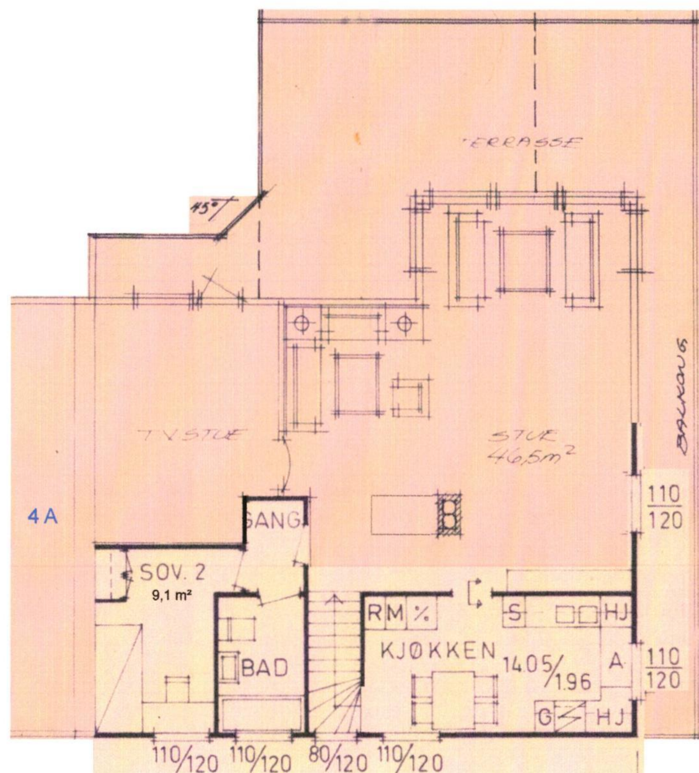
Plan 1. Etasje 1:100
