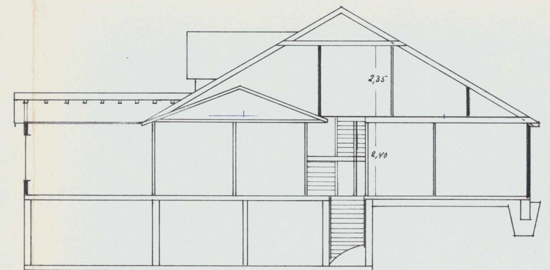
Snitt A-A
