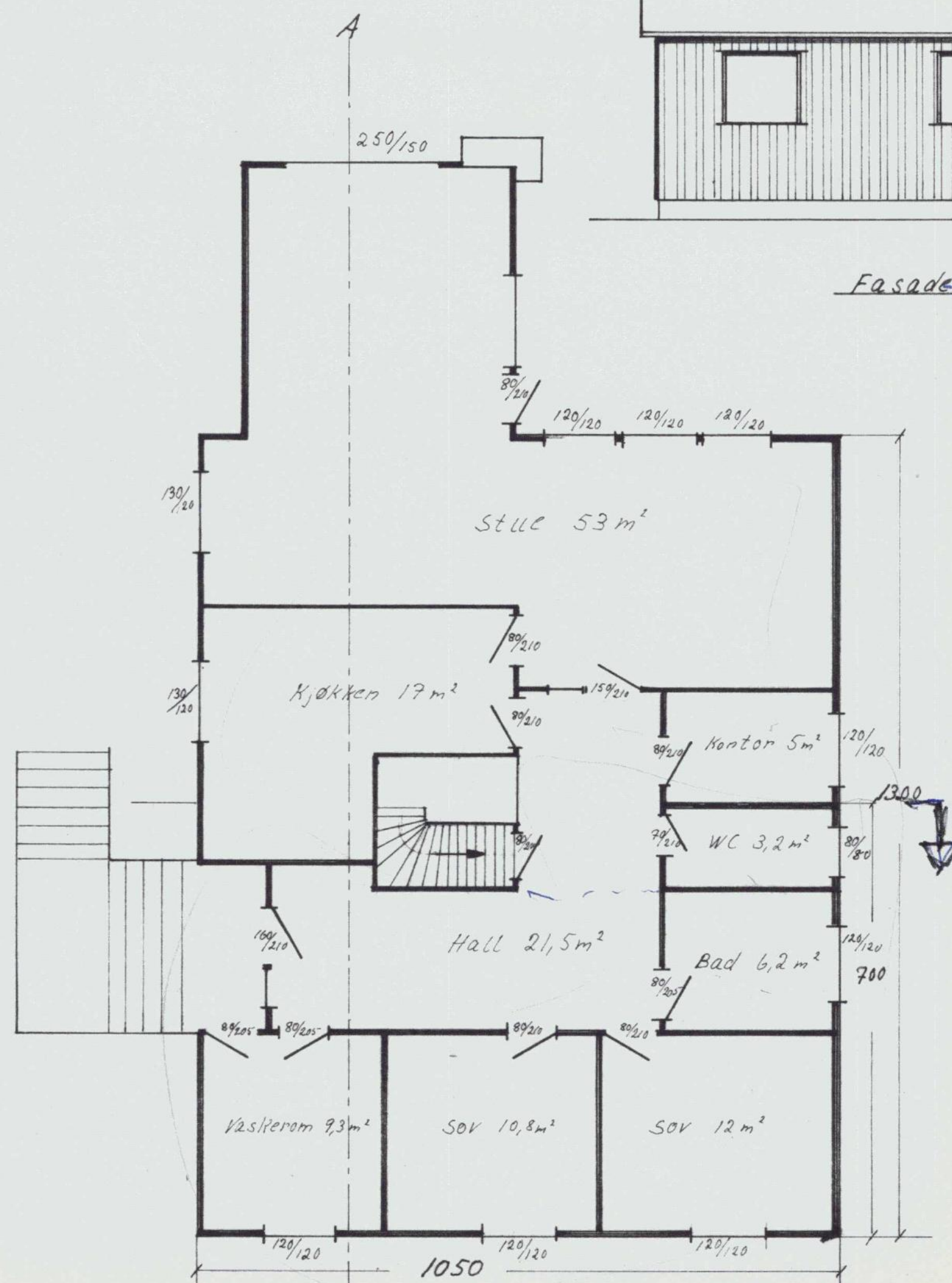
A Grunnplan I. etg.
