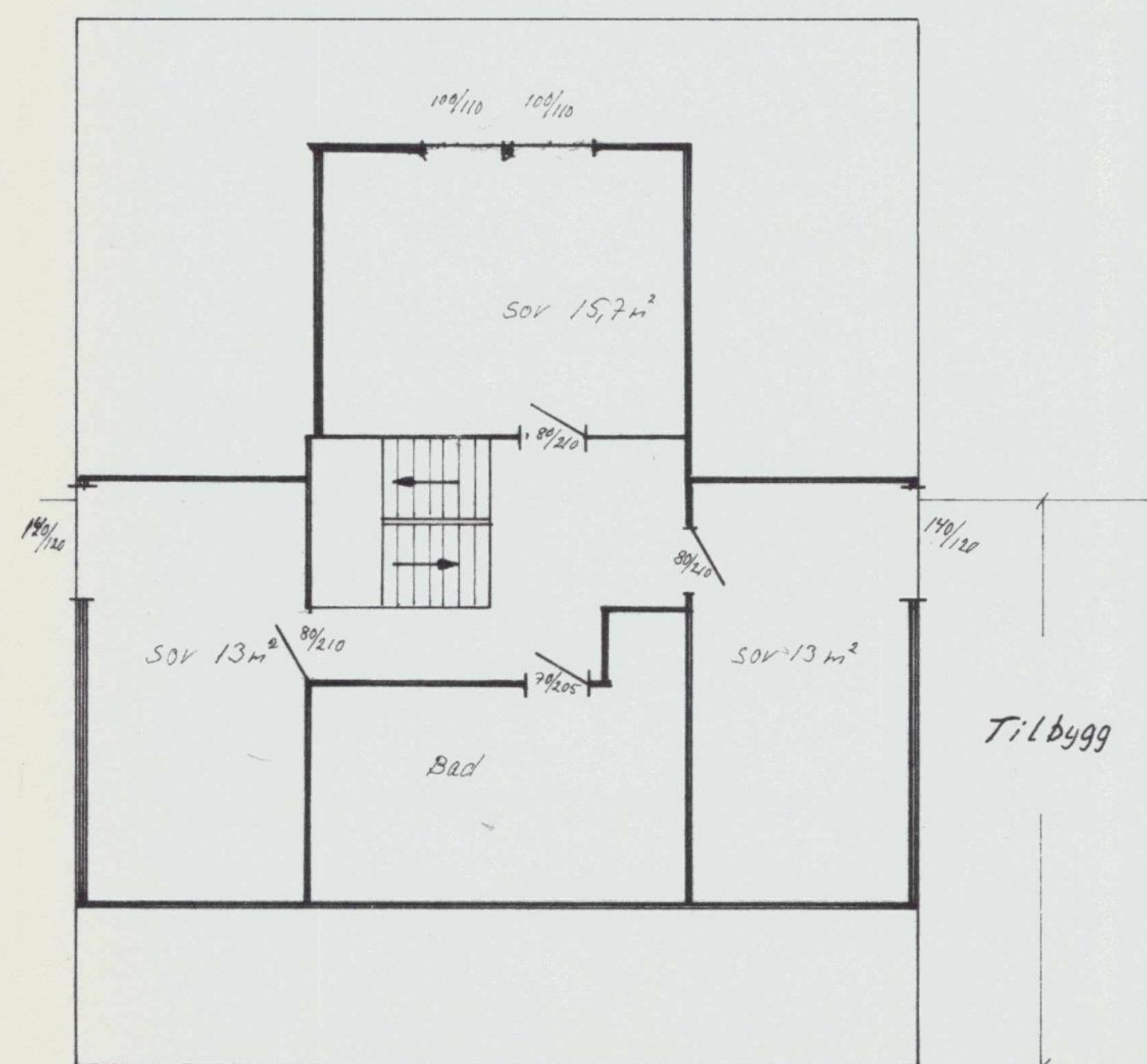
Grunnplan II. etg.
