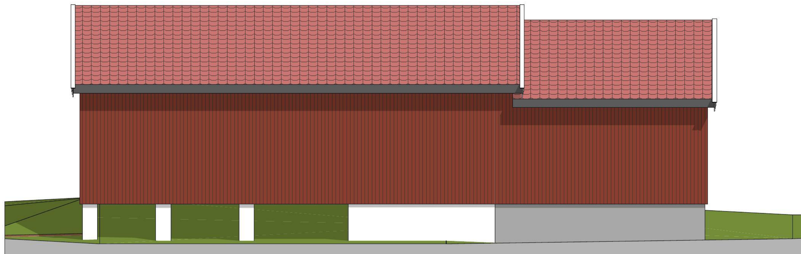
1:100 Fasade Vest
