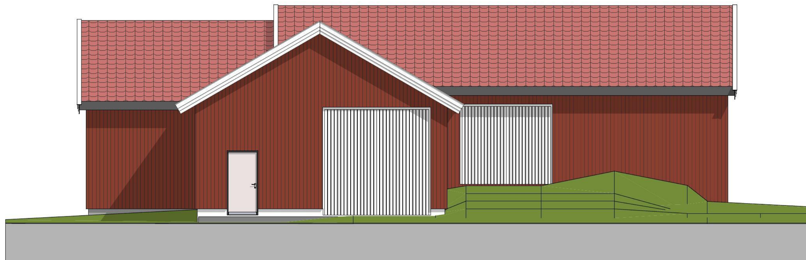
1:100 Fasade Øst
