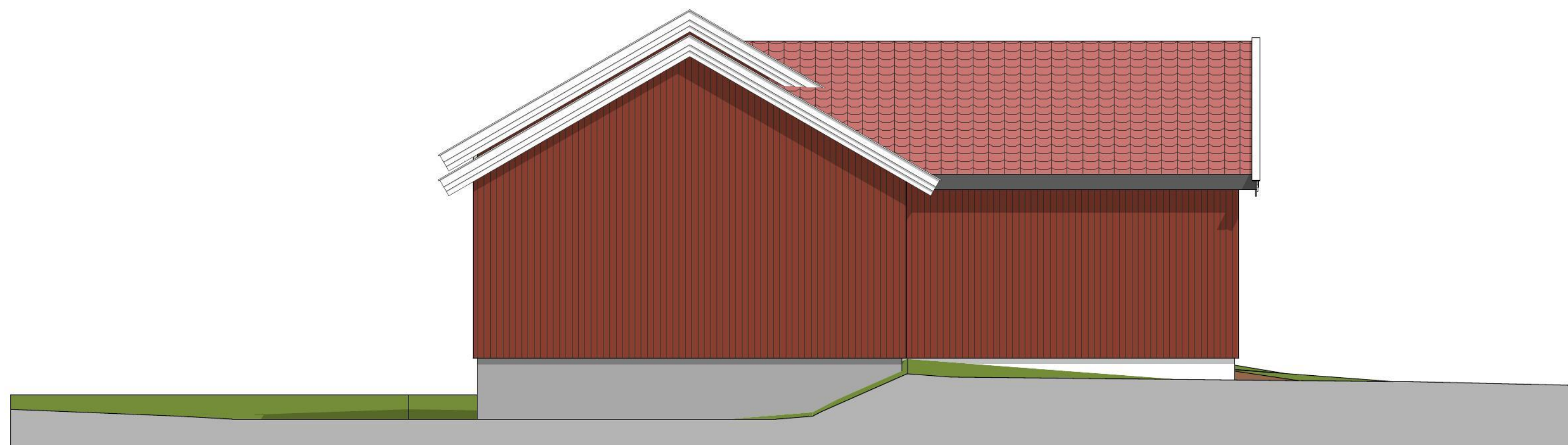
1:100 Fasade Sør
