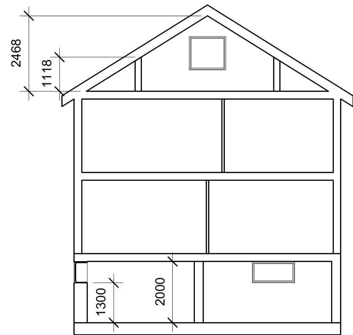
2 Snitt A 1 : 100
