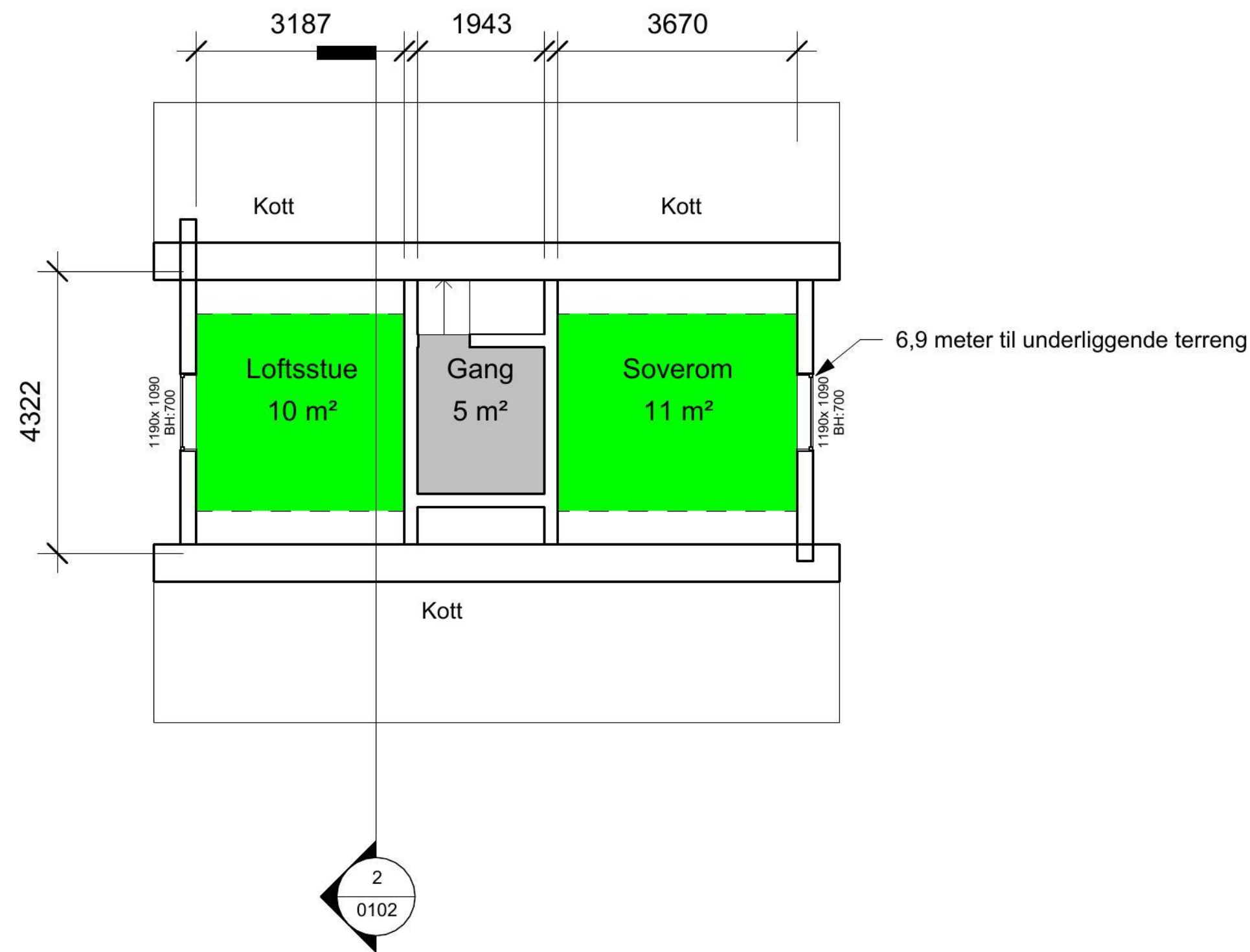
1 3. etasje 1 : 100
