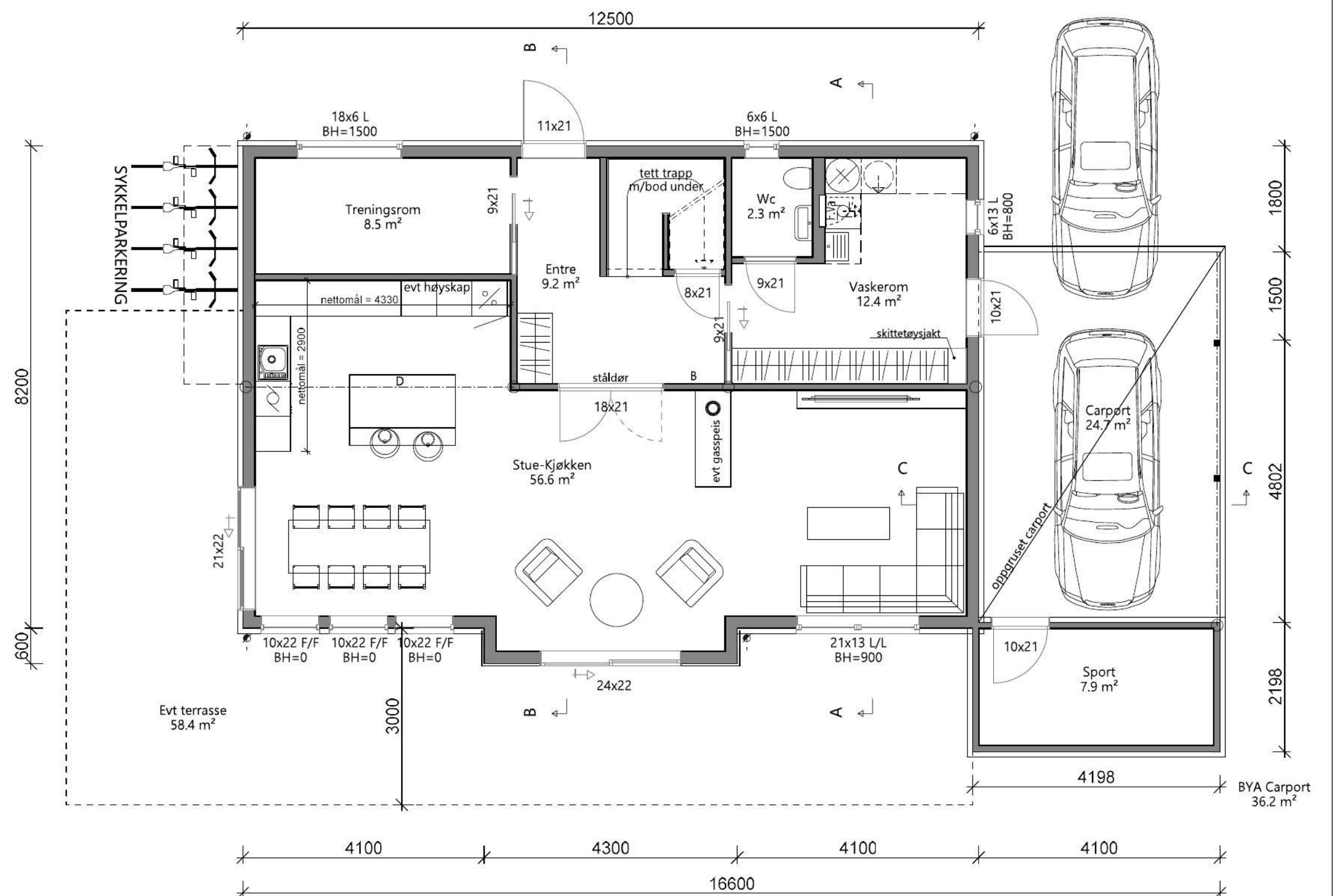
Plan 1. Etasje
