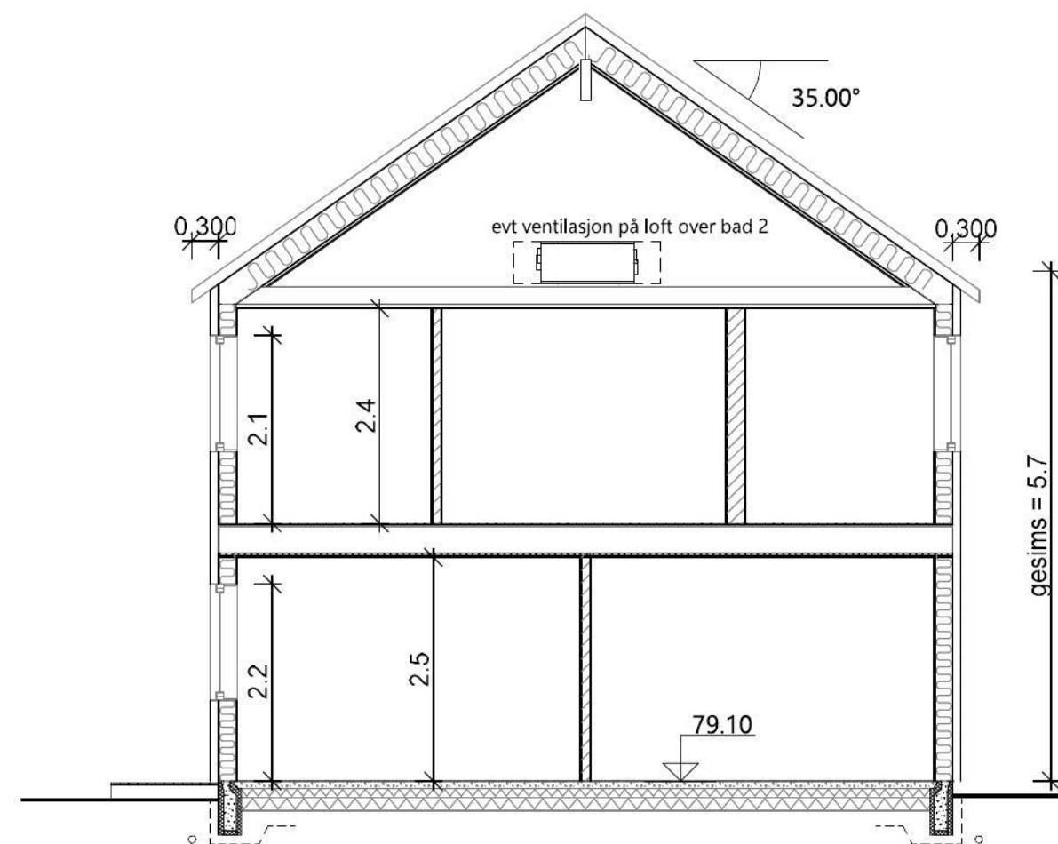
Snitt A-A
