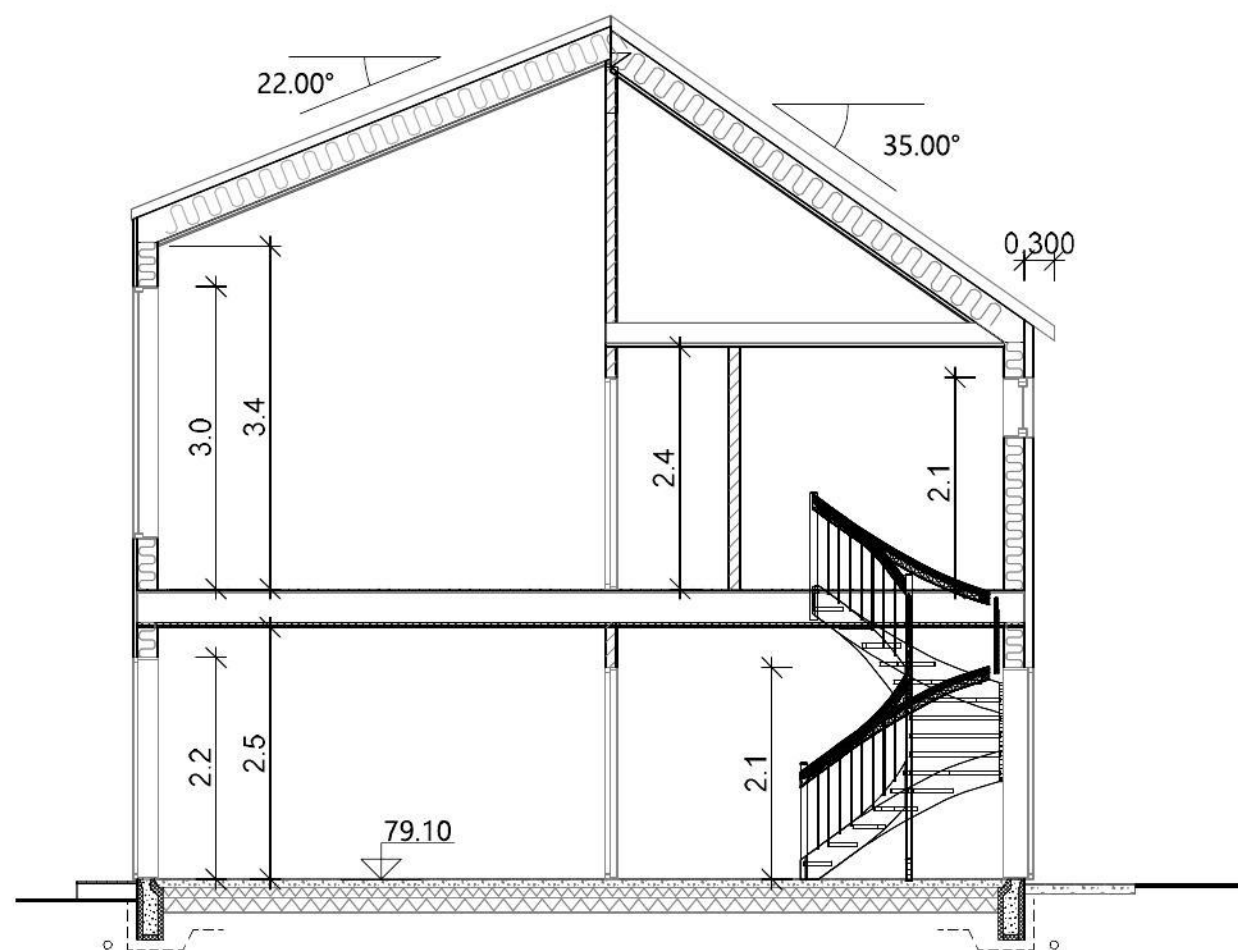
Snitt B-B
