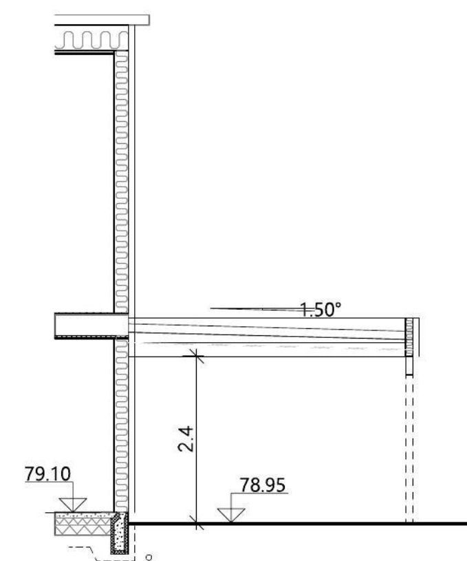
Snitt C-C
