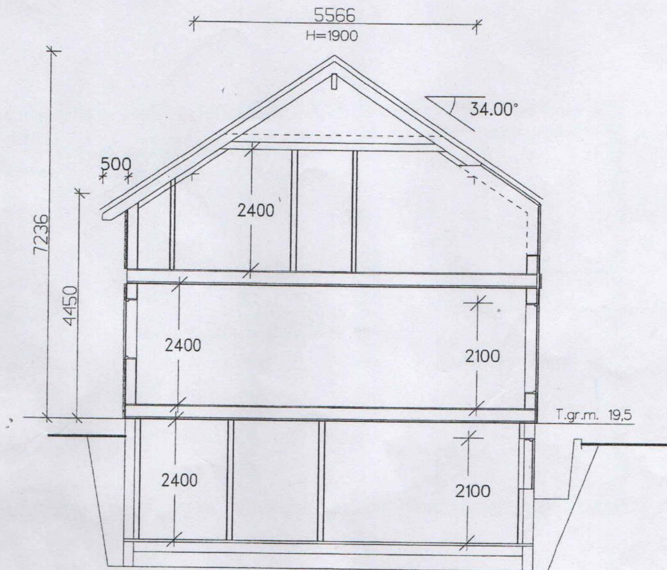
SNITT A-A
