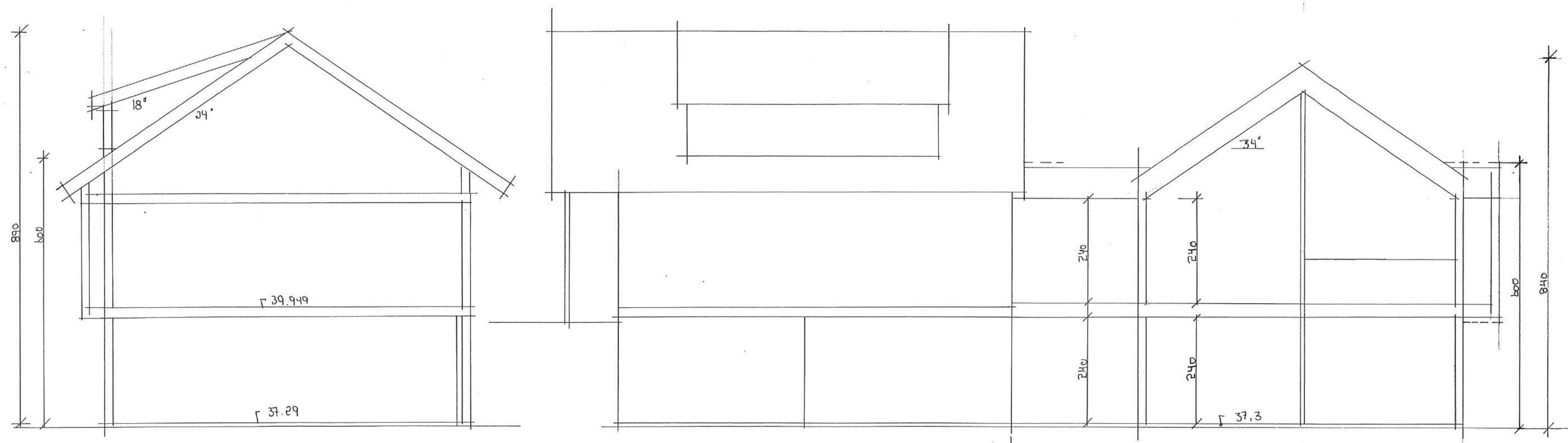
SNITT EKS. BOLIG
