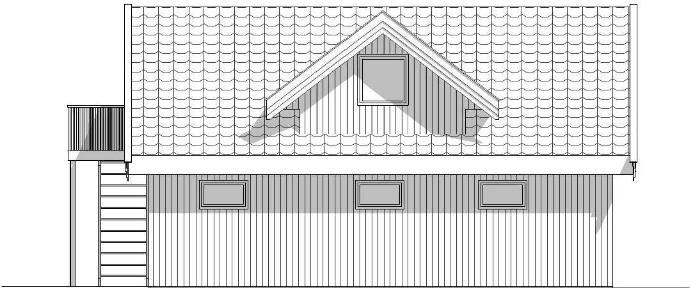
1:100 Fasade Vest
