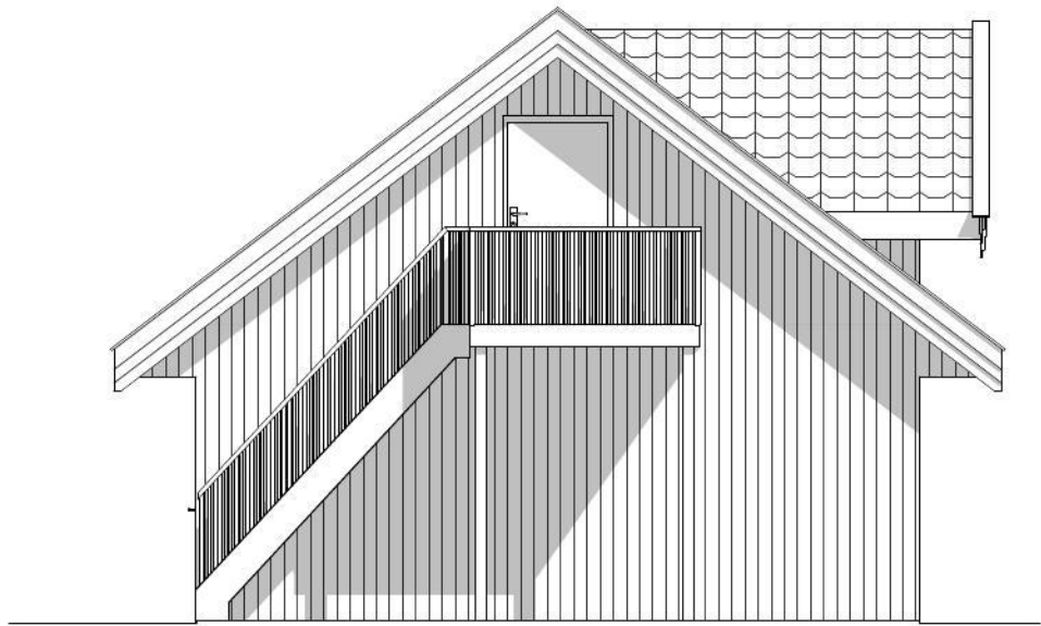
1:100 Fasade Nord
