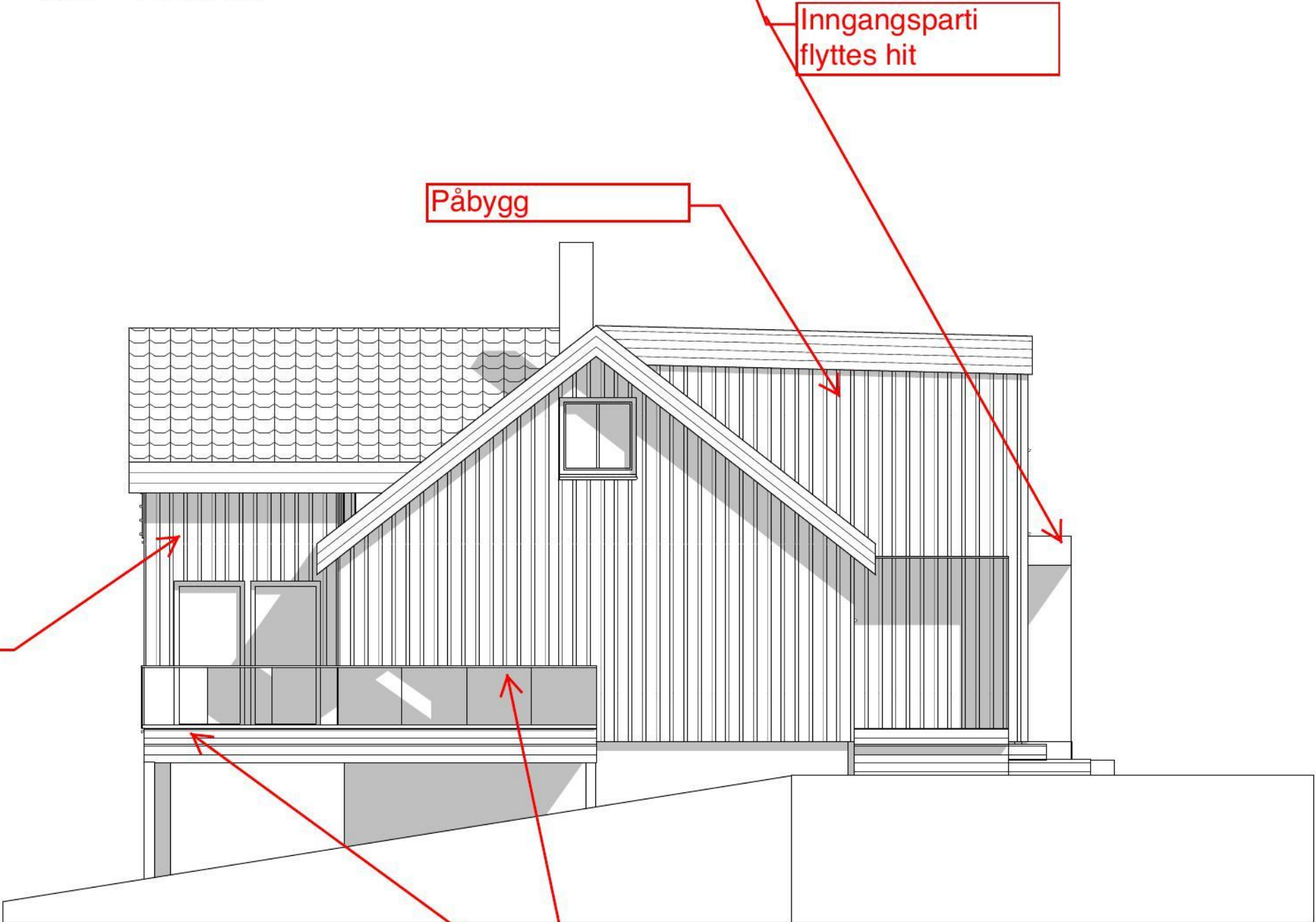
1:100 Fasade Sør
