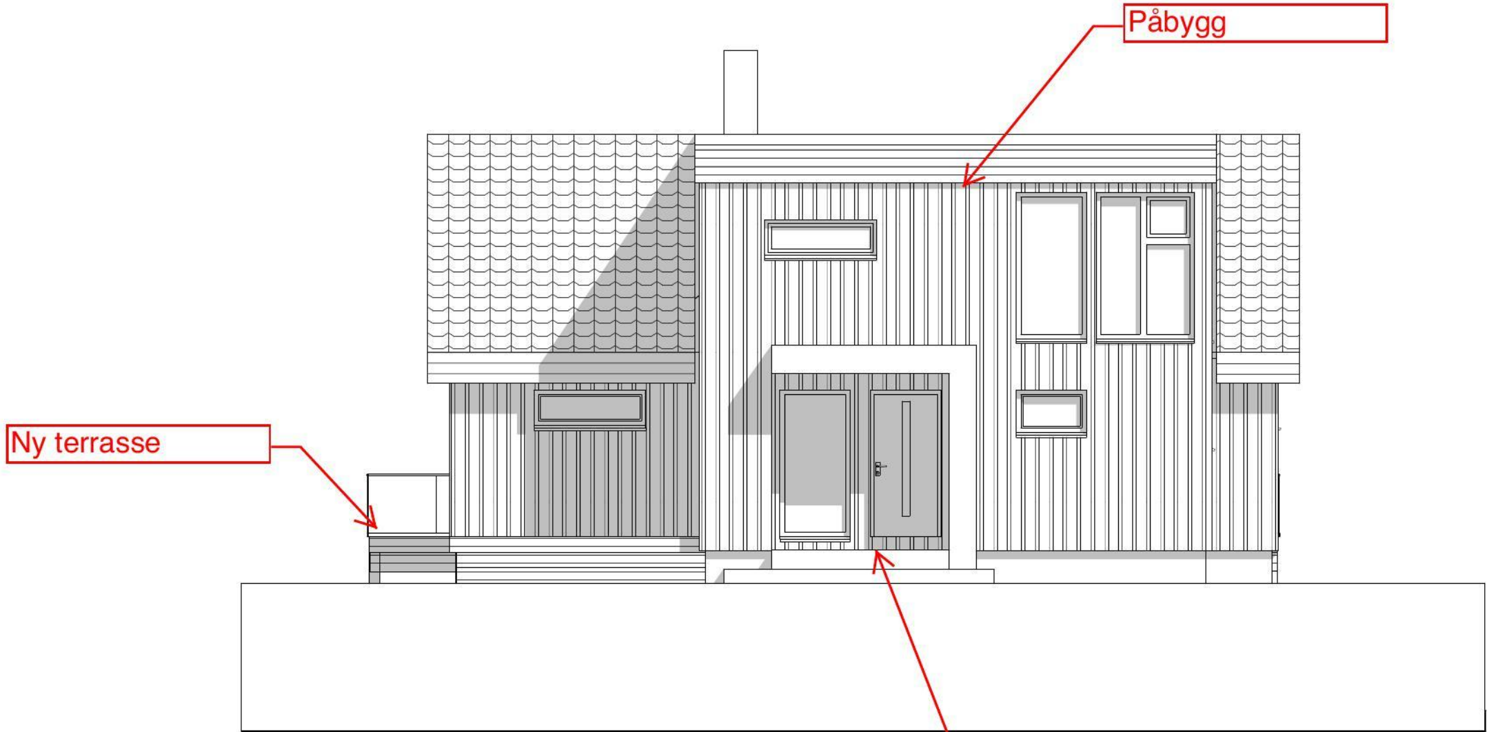
1:100 Fasade Øst
