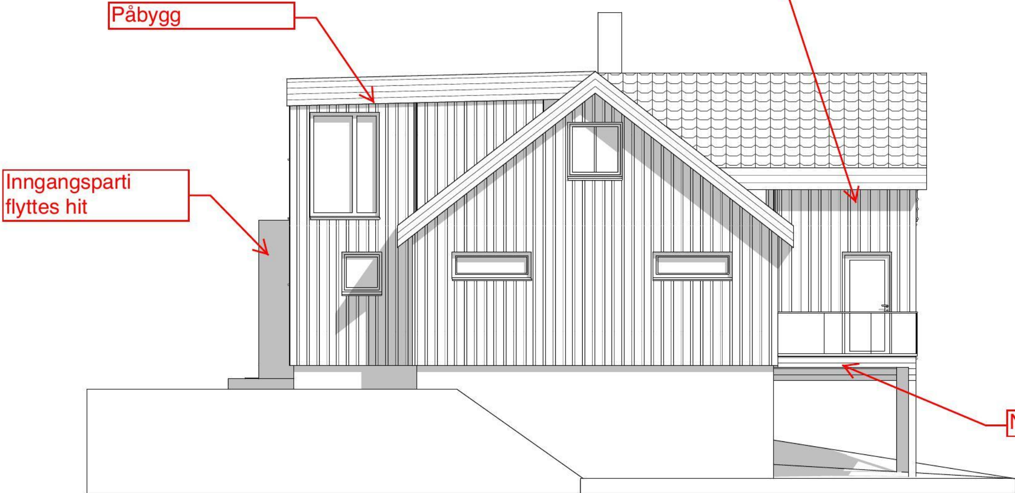
1:100 Fasade Nord
