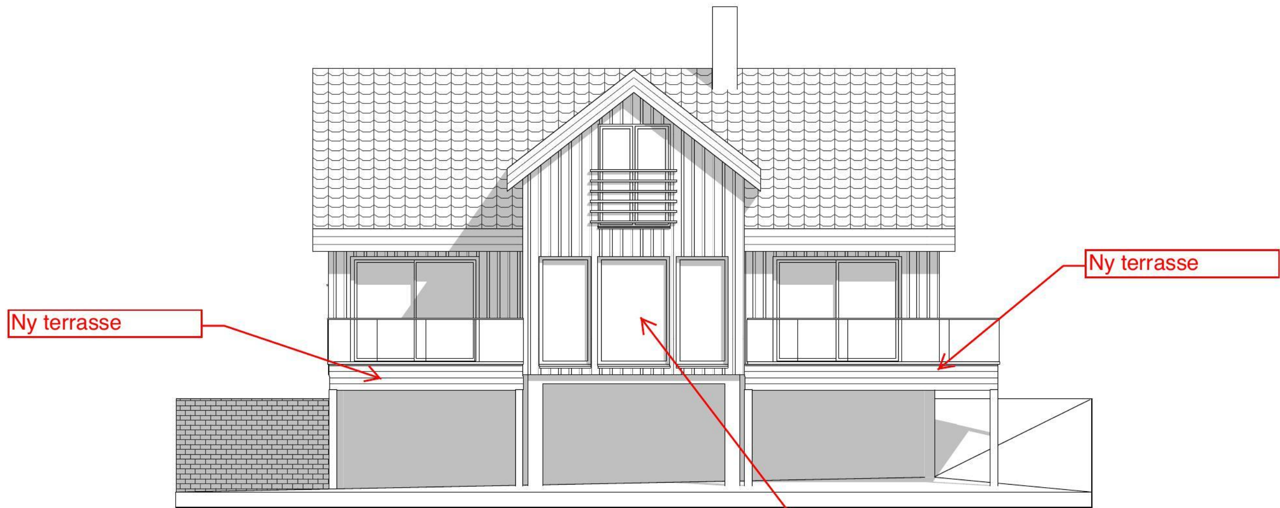
1:100 Fasade Vest
