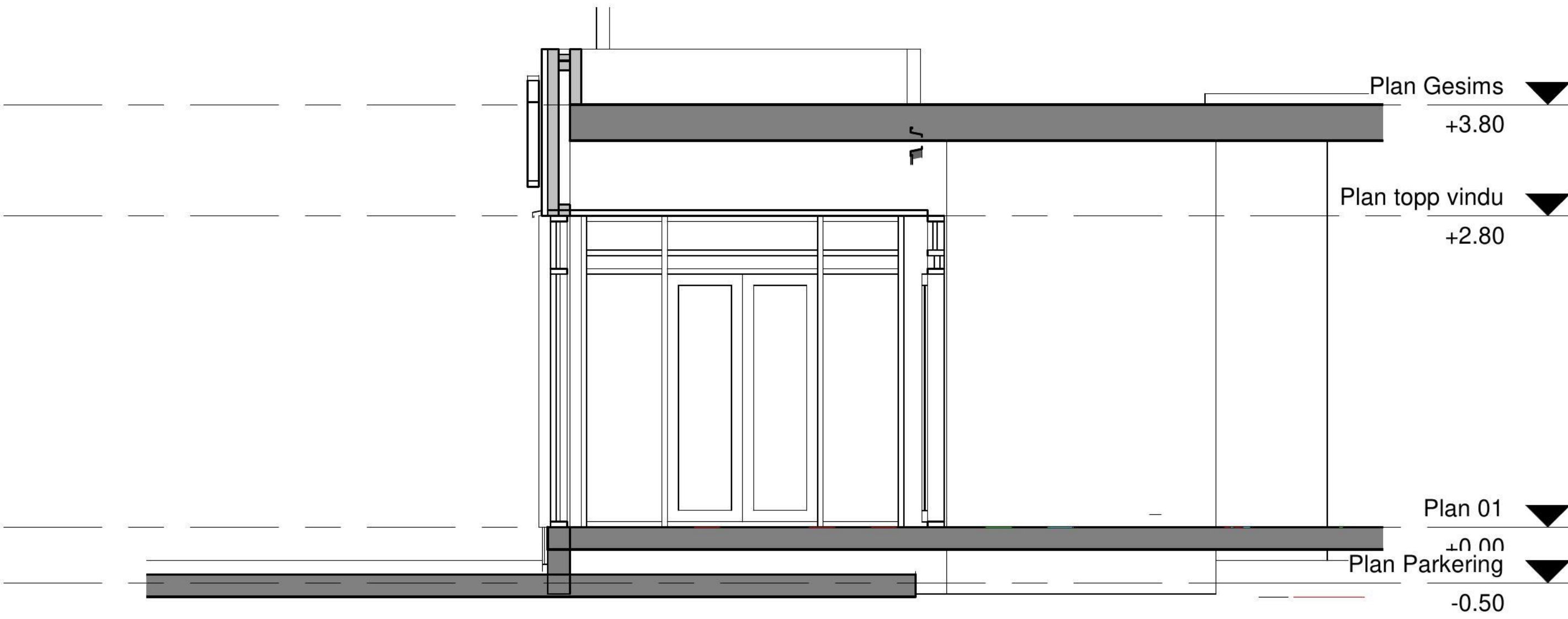
Fasade Sør 1 : 100
