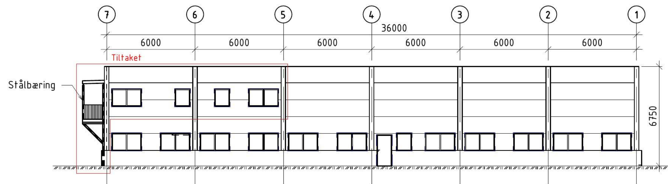
Fasade mot nord 1 : 200
