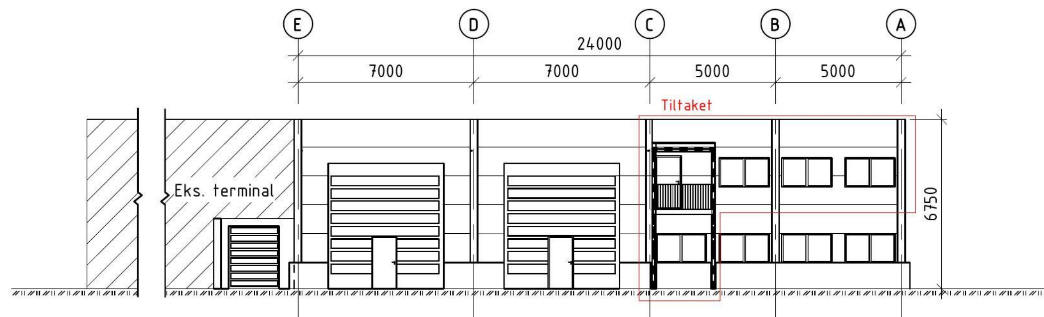
Fasade mot øst 1 : 200
