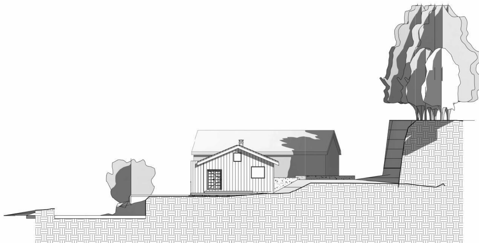
1 Nor-Vest 1 : 100
