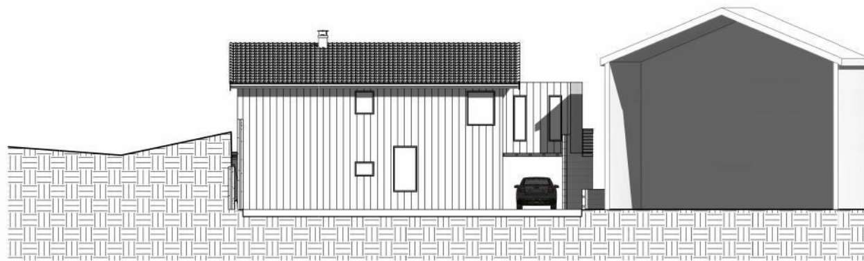
1 Sør-Vest 1 : 100
