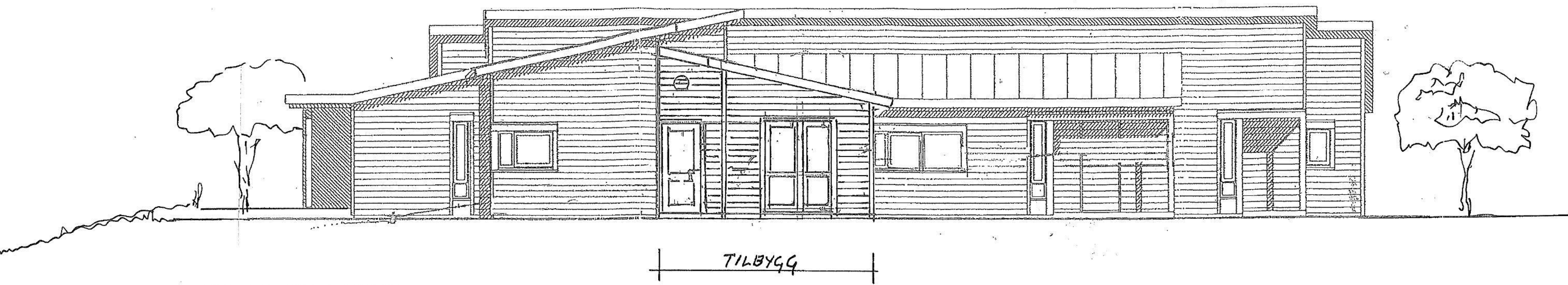
FASADE VEST
