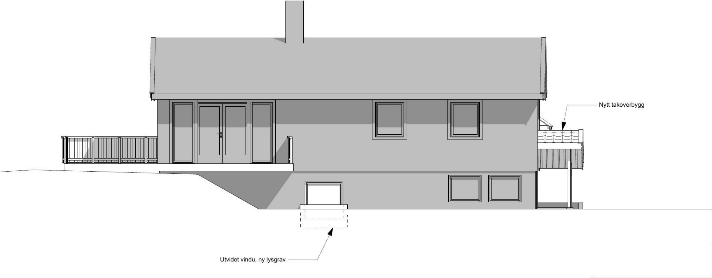
1:100 Fasade Sør
