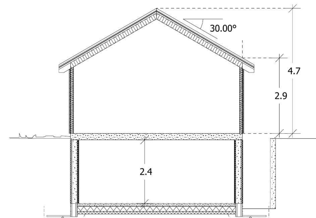
SNITT A-A
