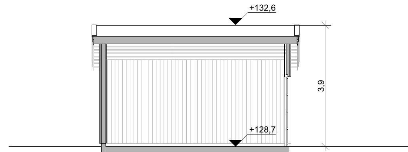
1:100 Snitt A
