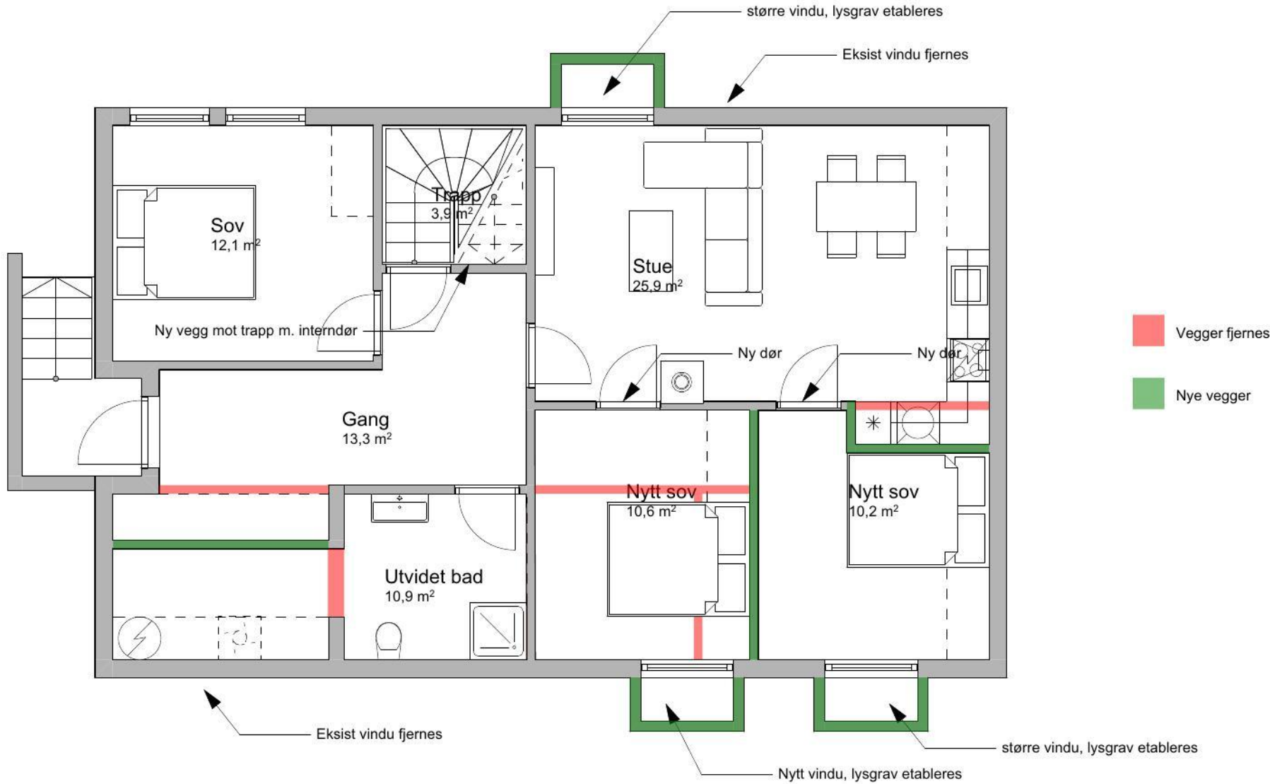
1:100 Kjeller ny
