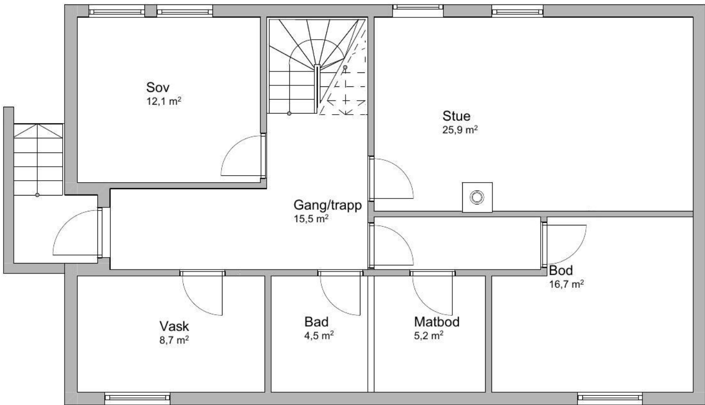
1:100 Kjeller eksist.
