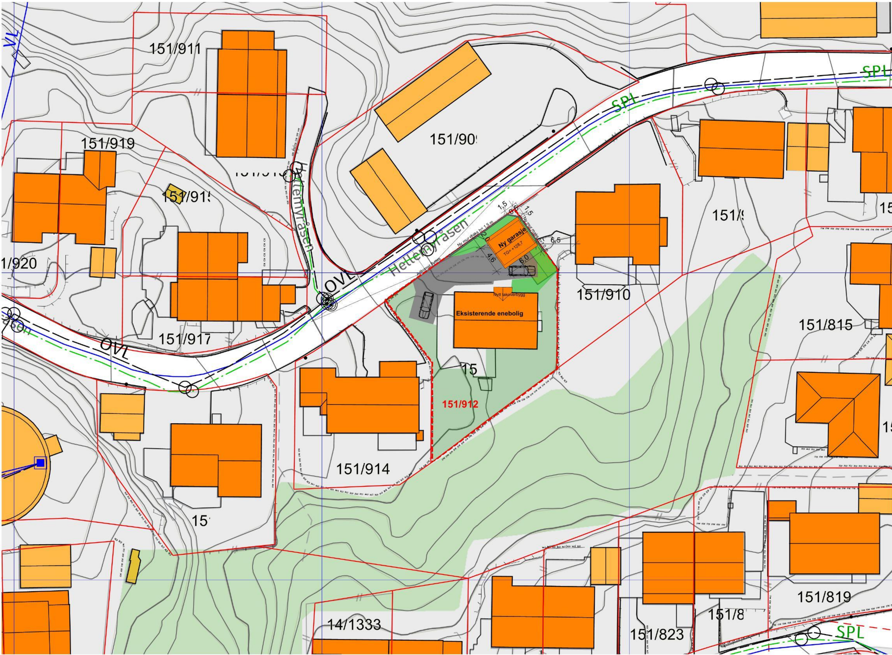
1:500 Situasjonsplan
