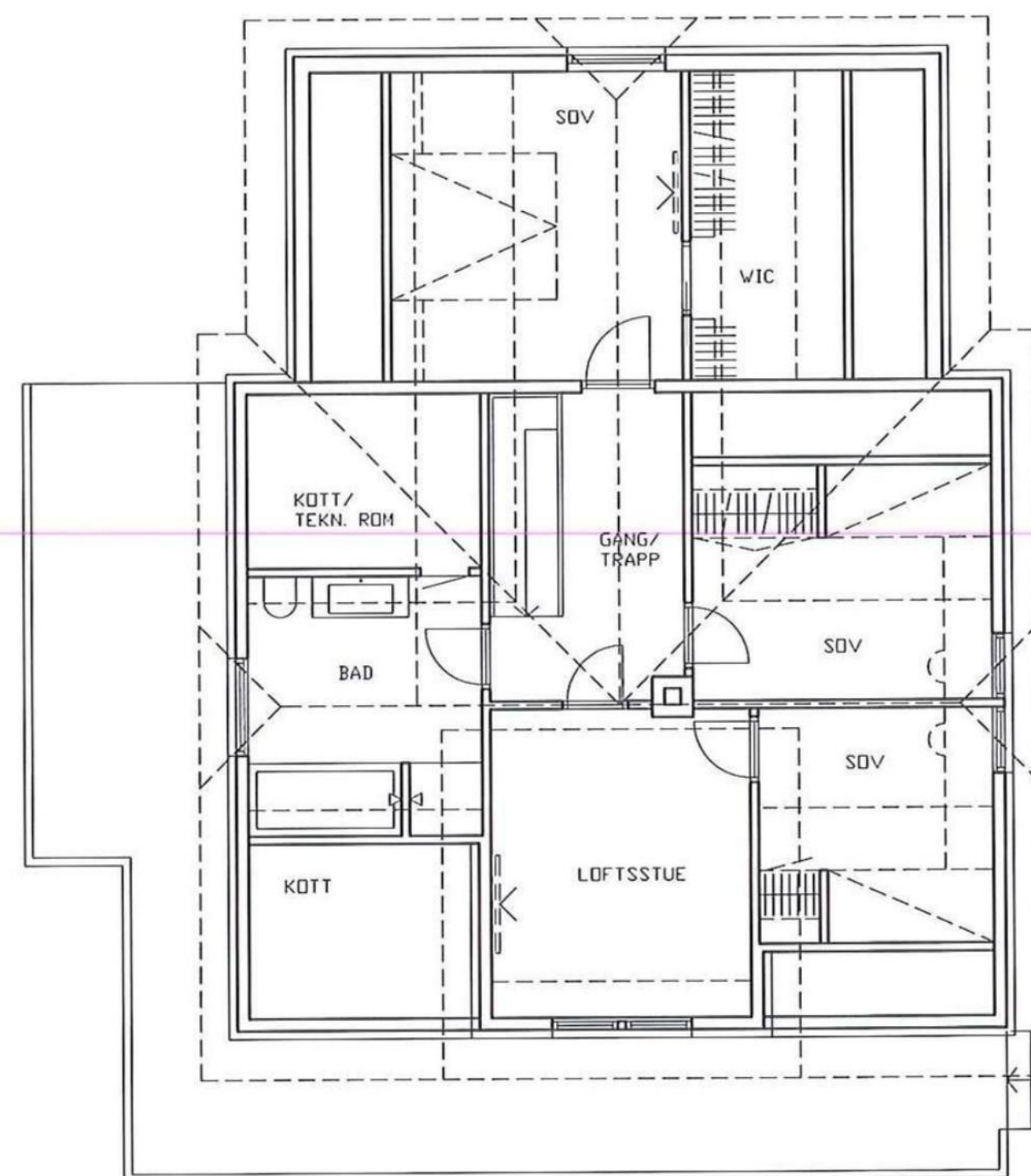
LOFT, ENDRINGSFORSLAG BRA 76,5 m 2
