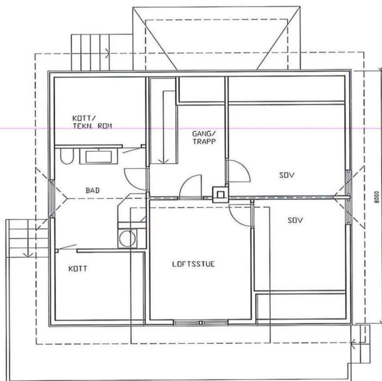
LOFT, EKSISTERENDE BRA 50,0 m 2
