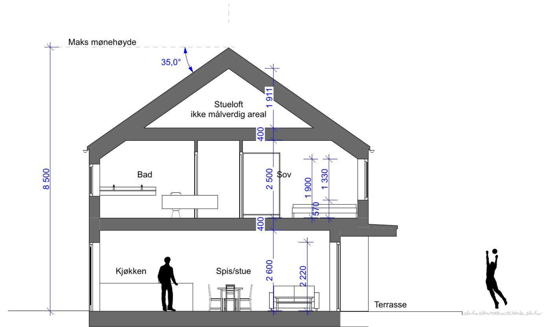
1:100 Snitt A
