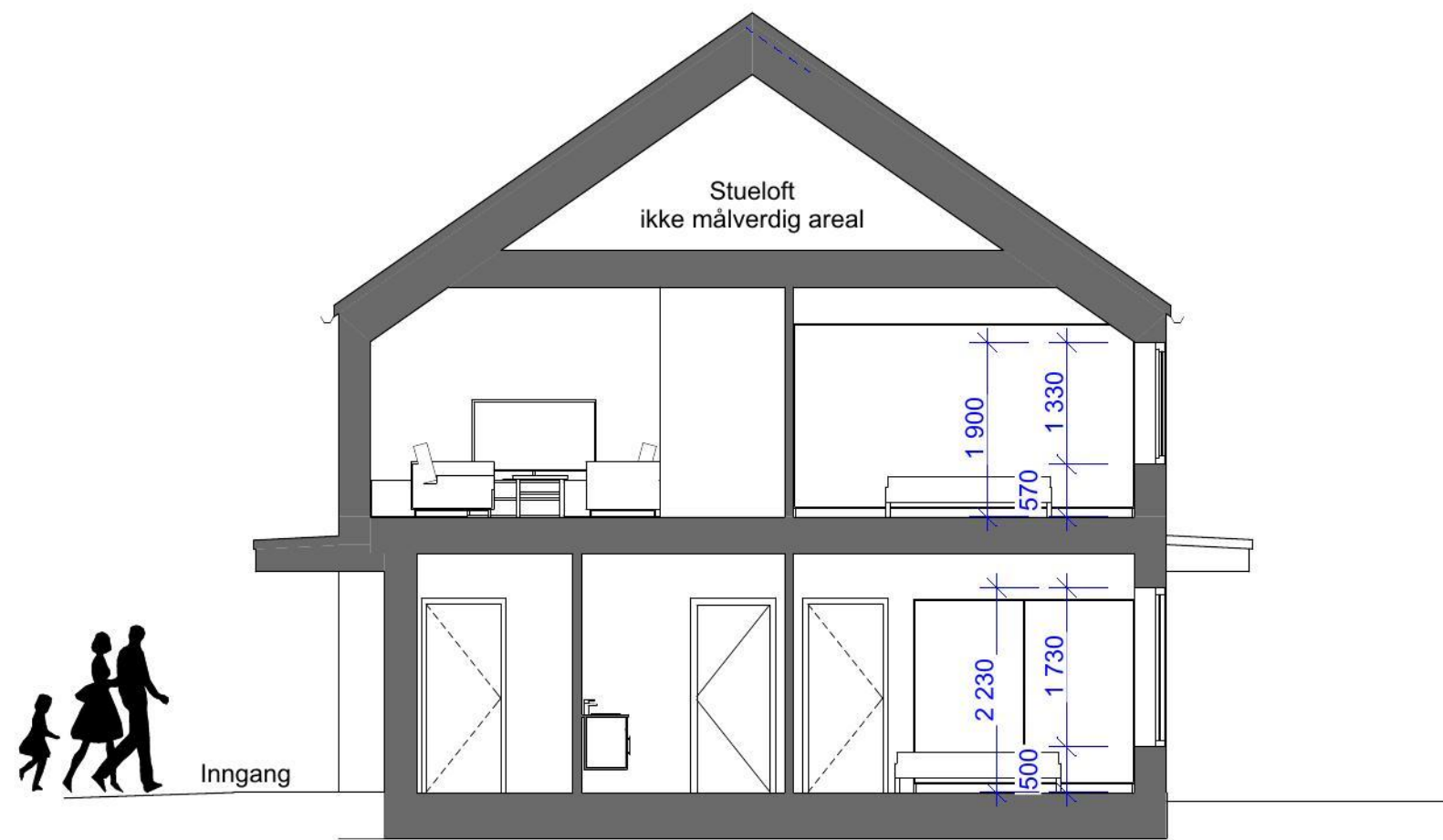
1:100 Snitt B
