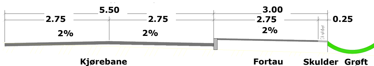
Figur 12. typisk normalprofil for veistrekningen.
