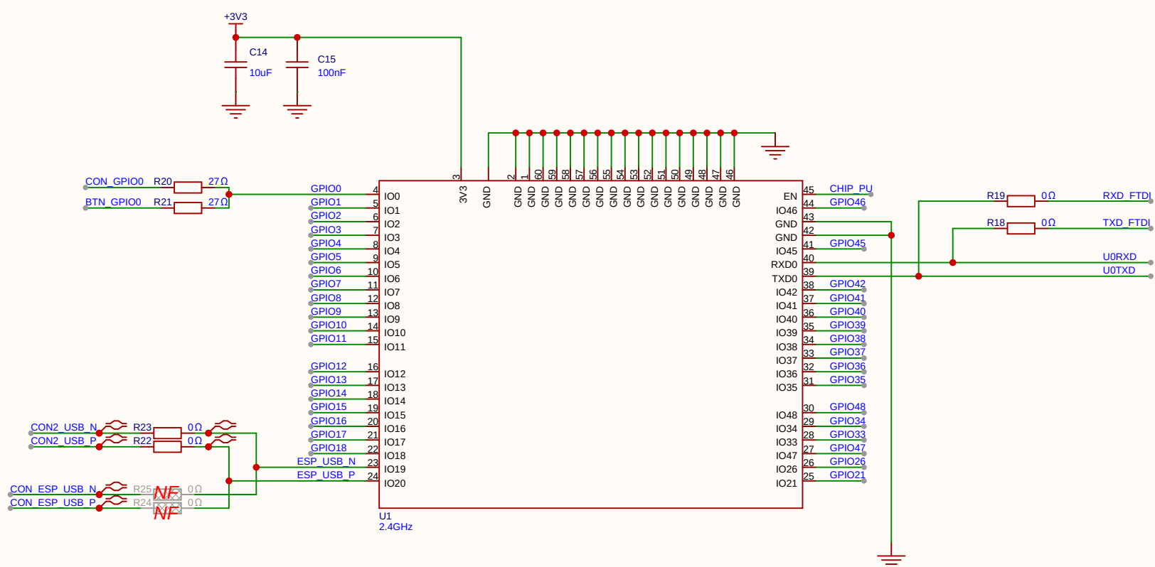
ESP32 MODULE
