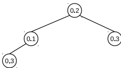
図: 葉の削除
