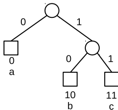
図: 符号の木
