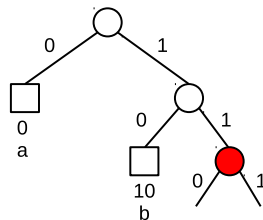
図: l_3 = 2 に対する節点の選択
