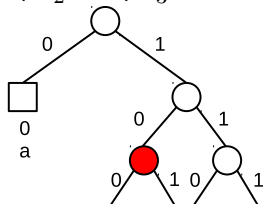
図: l_2 = 2 に対する節点の選択
