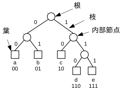
図: 符号の木
