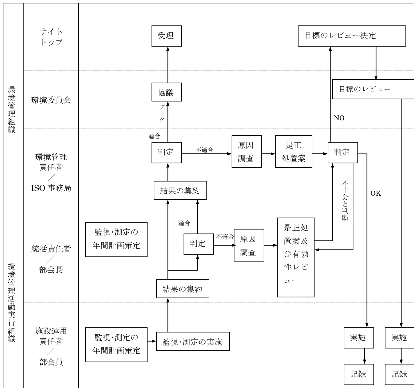
別表 26 (10.2) 監視・測定及び不適合是正処置のフロー
