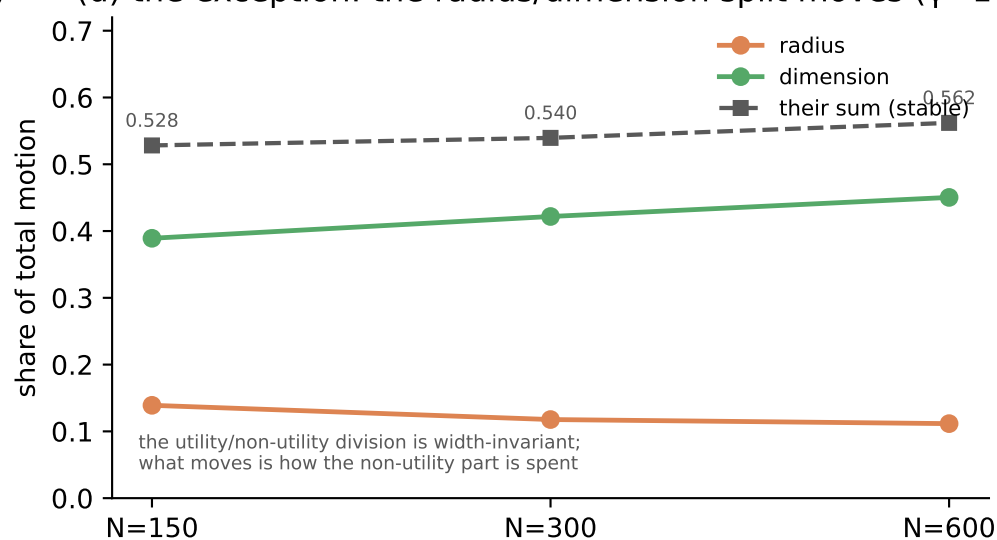
(d) the exception: the radius/dimension split moves ( \gamma=10 )
